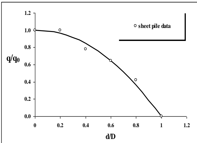
شکل ۵: اثر پرده آببند بر کاهش نشست
