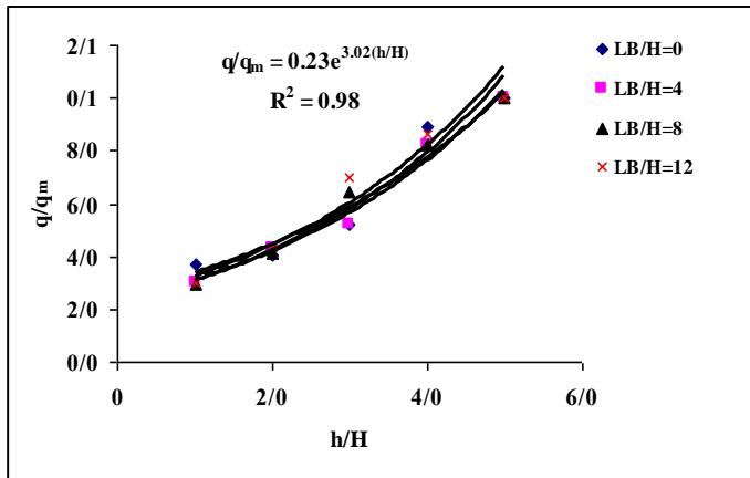
شکل ۹: اثر تراز آب بالادست بر میزان نشست برای نسبت d/D = 0.6
