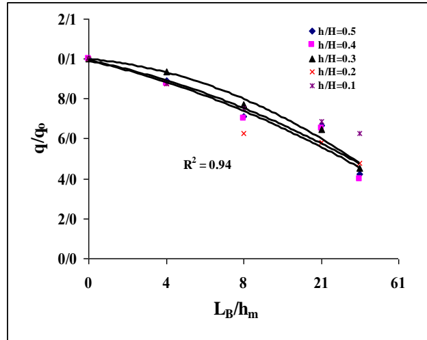
شکل ۴: اثر طول بلانکت بر میزان نشست بازای d/D = 0.2
