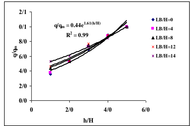
شکل ۷: اثر تراز آب بالادست بر میزان نشست برای نسبت d/D = 0.2
