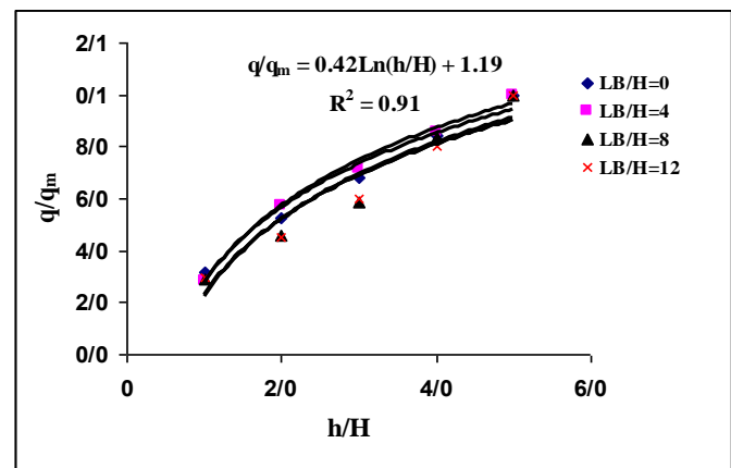
شکل ۸: اثر تراز آب بالادست بر میزان نشست برای نسبت d/D = 0.4
