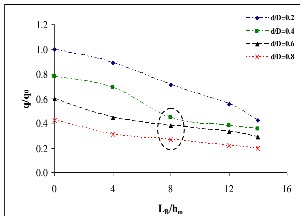
شکل شماره ۶: اثر تلفیقی بلانکت و پرده آب‌بند بر کاهش نشت در شرایط h/H = 0.5
