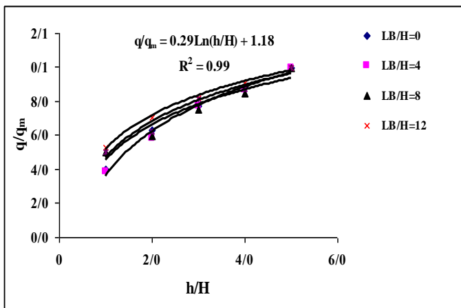
شکل ۱۰: اثر تراز آب بالادست بر میزان نشست برای نسبت d/D = 0.8
