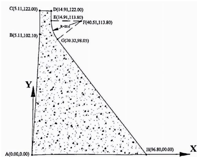
شکل ۱. مشخصات مقطع دوبعدی سد پاین فلت [۱۴] Fig. 1. Two-dimensional profile of Pine Flat Dam [14]
