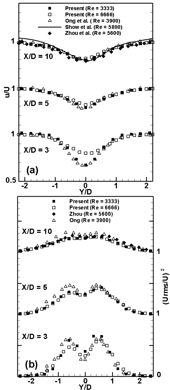
شکل (4): توزیع سرعت (شکل a) و میزان اغتشاش‌ها (شکل b) در فاصله 10 و 5 سیلندر دایره‌ای در اعداد رینولدز 3333 و 6666 و مقایسه با نتایج تجربی انگ و همکاران [3] و ژاو و همکاران [2] و عددی شاو و همکاران [4]
