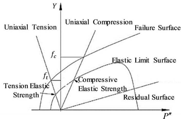
شکل ۱. سطوح حدی در مدل RHT [۲۹]
