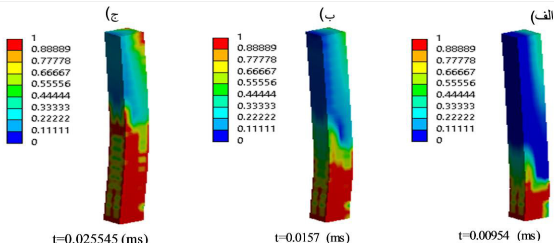
شکل ۹. کانتور تنش (شاخص خرابی) ستون در اثر انفجار ۷۲۹ کیلوگرم در فاصله سرد ۱۰ متر (الف) t=0.00954 (ب) t=0.0157 (ج) t=0.025545
