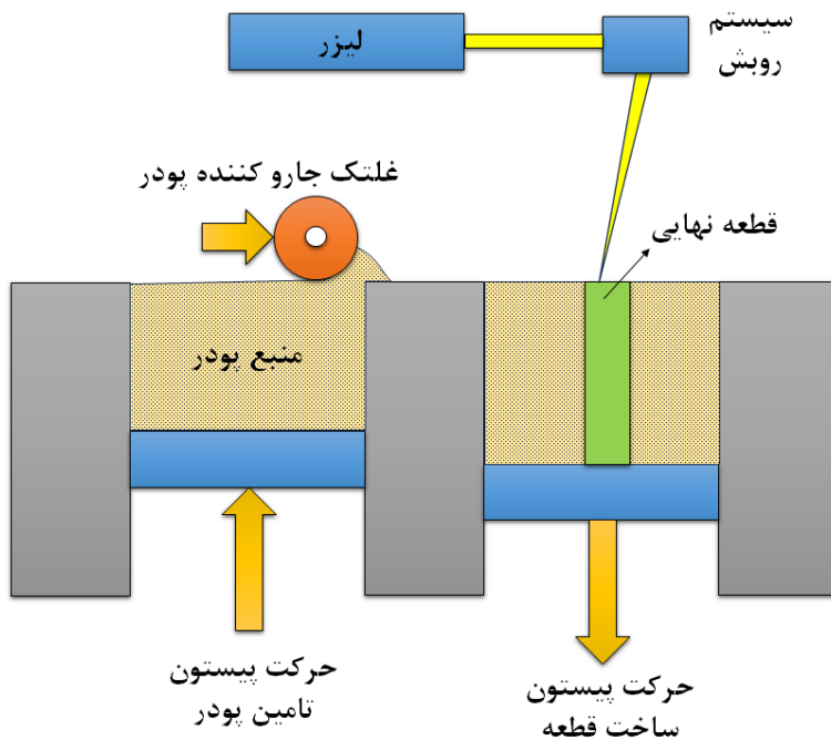
شکل ۱. شماتیک نشان دهنده روش ساخت قطعات اولیه به کمک روش ذوب لیزری انتخابی.
