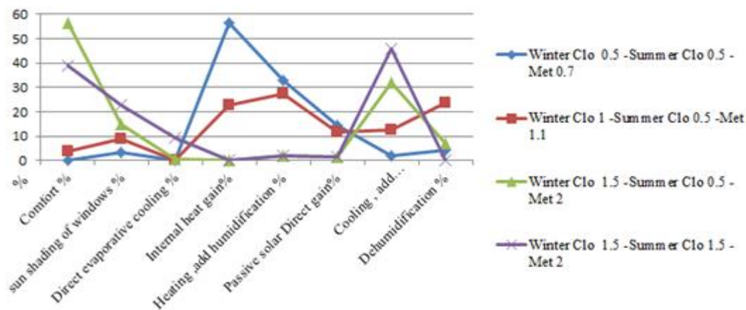
شکل ۱۰. نتایج پارامترهای فعال و غیرفعال در کلوها و میت مختلف در اقلیم sfa
