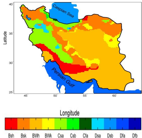
شکل ۱. طبقه‌بندی اقلیم کوپن - گایگر در ایران [۱۷]
