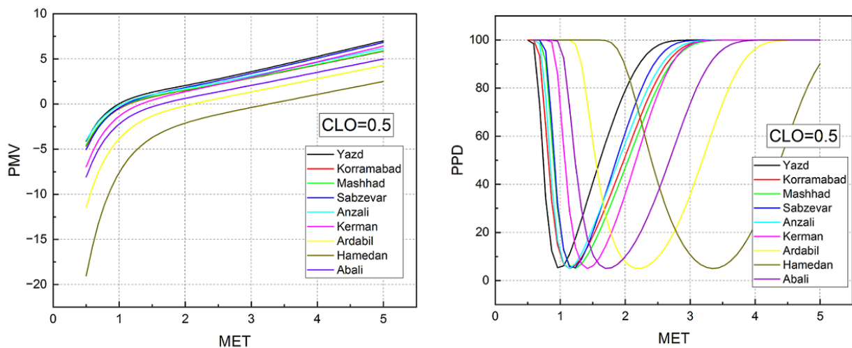
شکل ۱۳. نمودار پیاموی و پیبیدی در کلوی ۰/۵ برای ۹ اقلیم ایران
