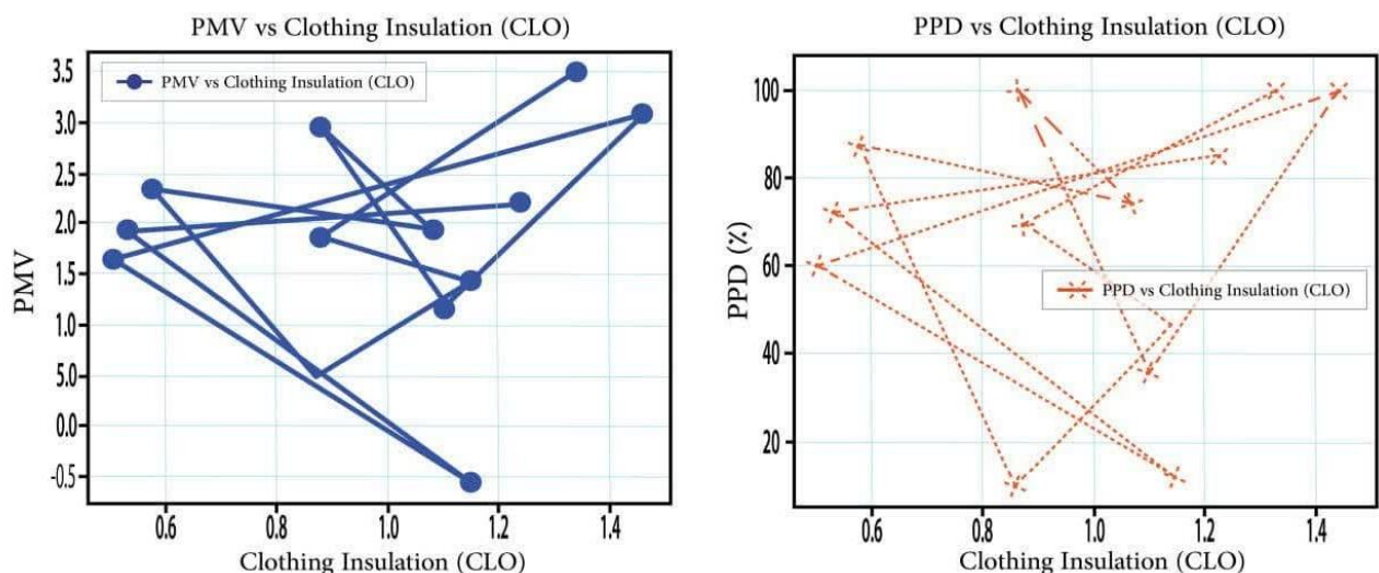
شکل ۷. نتایج آسایش حرارتی پی‌ام‌وی و پی‌پی‌دی در مقابل کلو
