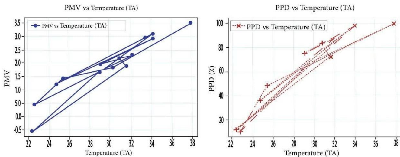
شکل ۳. نتایج آسایش حرارتی مدل پی ام وی و پی پی دی در مقابل دما
