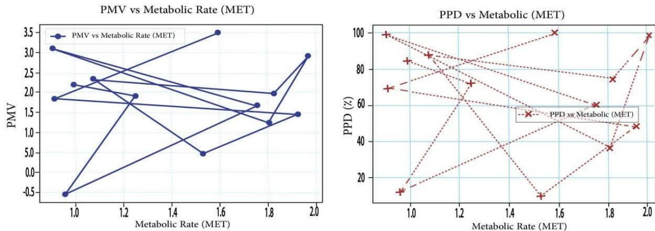
شکل ۶. نتایج آسایش حرارتی پی‌ام‌وی و پی‌پی‌دی در مقابل میت
