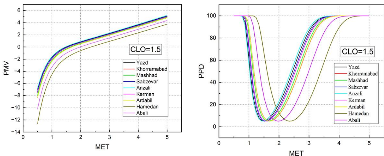
شکل ۱۴. نمودار پی‌ام‌وی و پی‌بی‌دی در کلوی ۱/۵ برای ۹ اقلیم ایران
