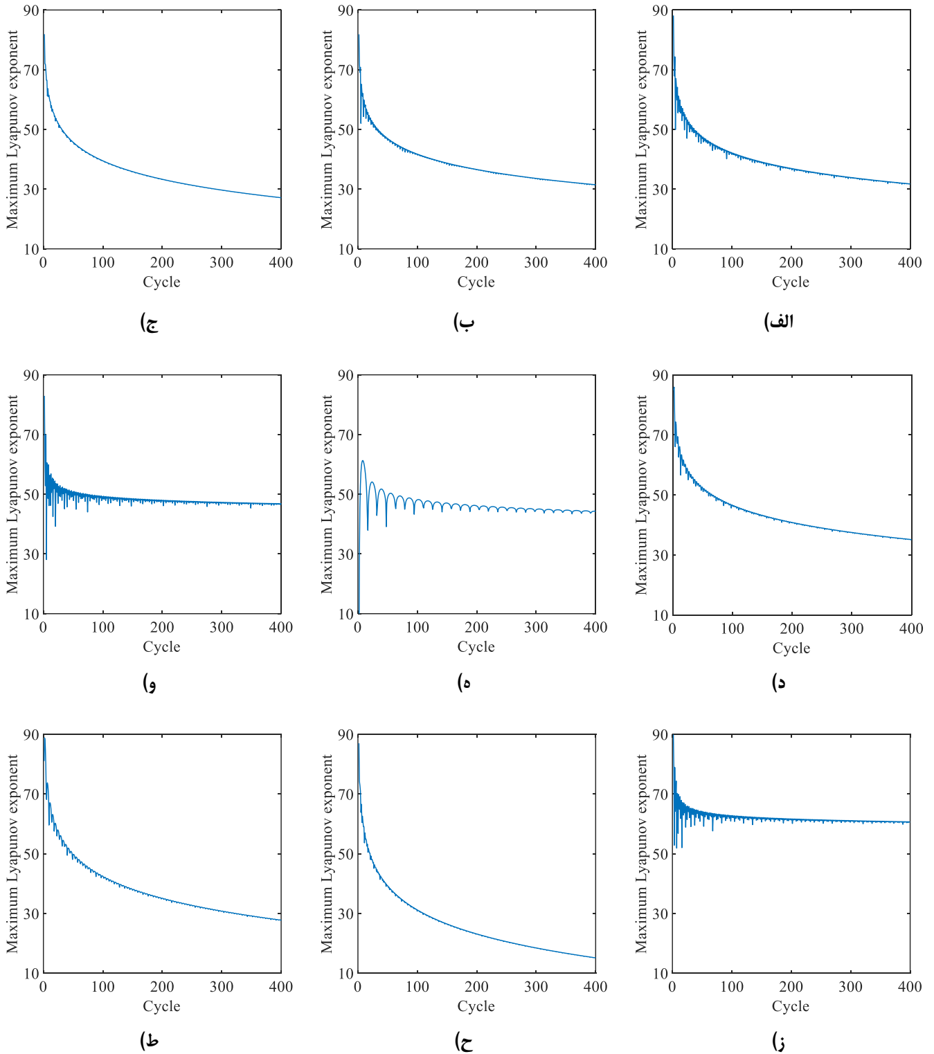
شکل ۸. ماکزیمم نمای لیاپانوف سیستم به ازای مقادیر (الف) R=100\text{ k}\Omega , \omega/2\pi=11\text{ Hz} (ب) R=100\text{ k}\Omega , \omega/2\pi=15\text{ Hz} (ج) R=100\text{ k}\Omega , \omega/2\pi=21\text{ Hz} (د) R=100\text{ k}\Omega , \omega/2\pi=34\text{ Hz} (ه) R=340\text{ k}\Omega , \omega/2\pi=16\text{ Hz} (و) R=340\text{ k}\Omega , \omega/2\pi=30\text{ Hz} (ز) R=340\text{ k}\Omega , \omega/2\pi=55\text{ Hz} (ح) R=500\text{ k}\Omega , \omega/2\pi=10.5\text{ Hz} (ط) R=500\text{ k}\Omega , \omega/2\pi=58\text{ Hz} (ی) R=500\text{ k}\Omega , \omega/2\pi=58\text{ Hz} .
