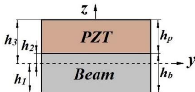
شکل ۲. مقطع عرضی تیر و لایه پیزوالکتریک
