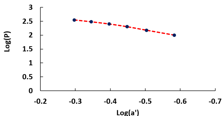
شکل ۵. نمودار \log(P) - \log(a') برای نمونه آزمایش شده.
