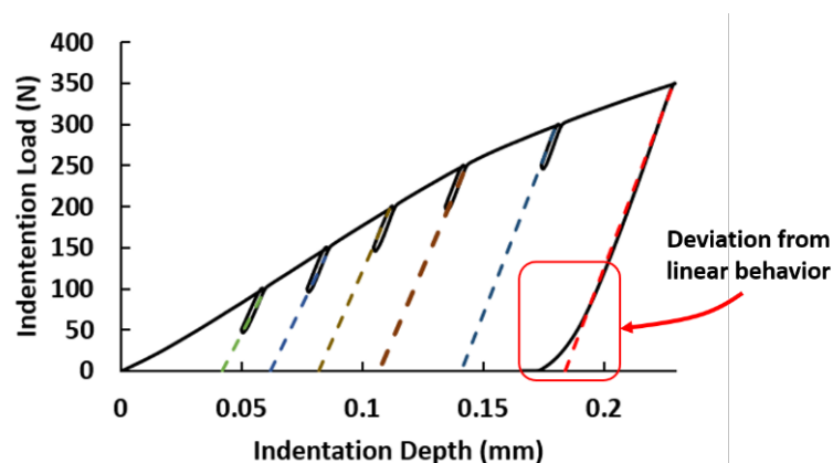
شکل ۴. نمودار بار-عمق نفوذ اندازه‌گیری شده و برازش خطی بخش اولیه نمودار باربرداری.
