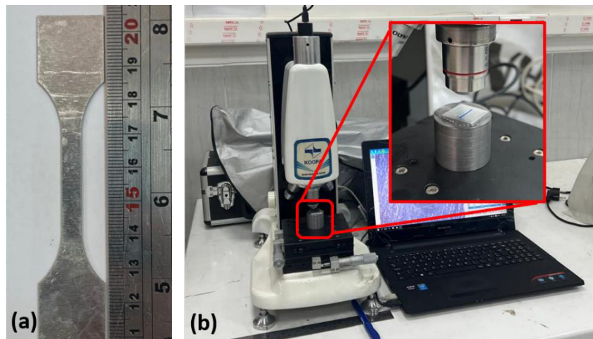
شکل ۱. نمونه‌های آزمایش آماده شده: (الف) نمونه کشش، (ب) نمونه فروری.
