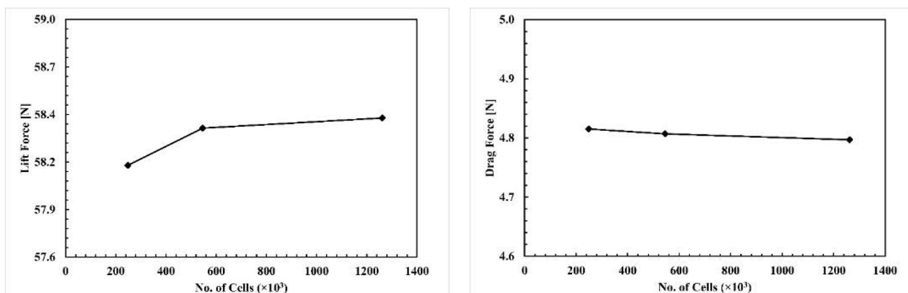
شکل ۵. مطالعه استقلال از شبکه نمونه پایه ایرفویل ناکا ۰۰۱۲ در فرکانس چرخش ۵ هرتز.
