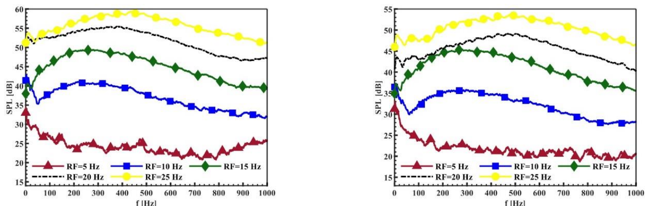
شکل ۱۴. مقایسه توزیع میانگین نمودارهای سطح فشار صوت در فرکانس‌های نوسانی مختلف برای میکروفون به فاصله ۱۰ متری از طول وتر ایرفویل ناکا ۰۰۱۲ (سمت چپ) مدل پایه و سمت راست) مدل با دندان. .
