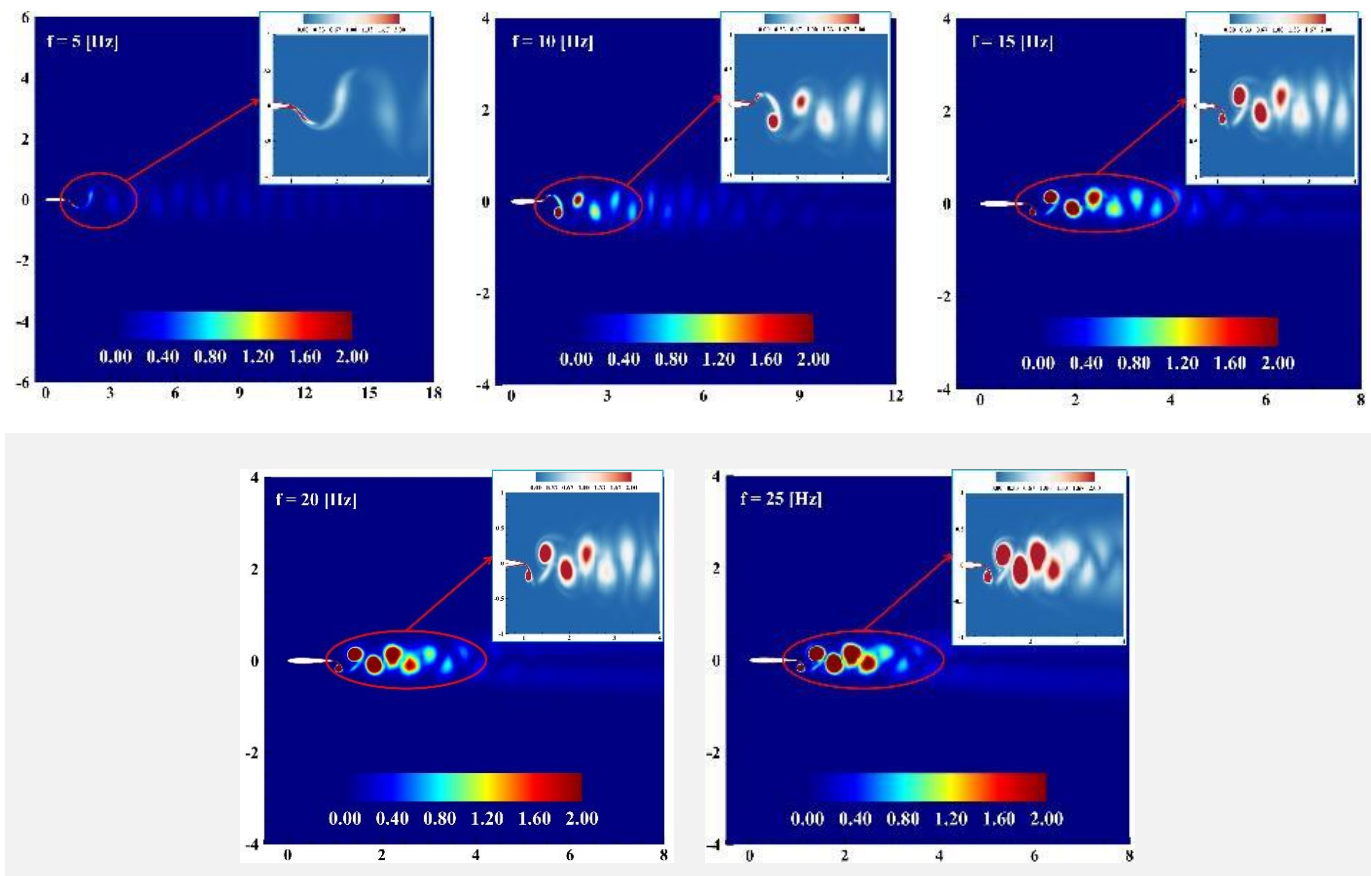
شکل ۹. خطوط هم‌مرز چرخش بی‌بعد برای مدل پایه ایرفویل ناکا ۰۰۱۲ در فرکانس‌های چرخش به ترتیب از چپ به راست ۵، ۱۰، ۱۵، ۲۰ و ۲۵ هرتز.
