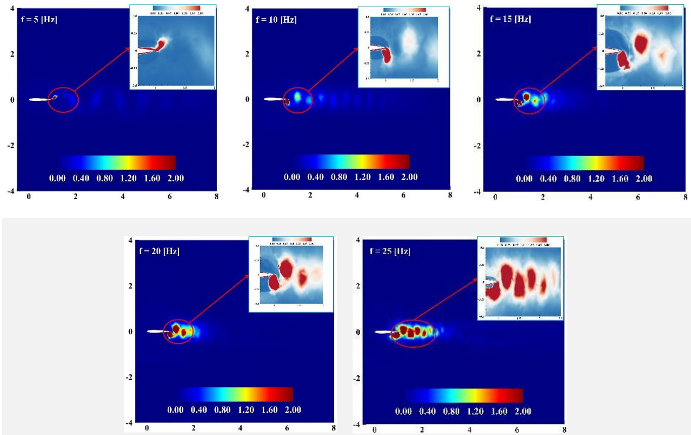
شکل ۱۰. خطوط هم‌مرز چرخش بی‌بعد برای مدل با دندان‌های ایرفویل ناکا ۰۰۱۲ در فرکانس‌های چرخش به ترتیب از چپ به راست ۵، ۱۰، ۱۵، ۲۰ و ۲۵ هرتز.
