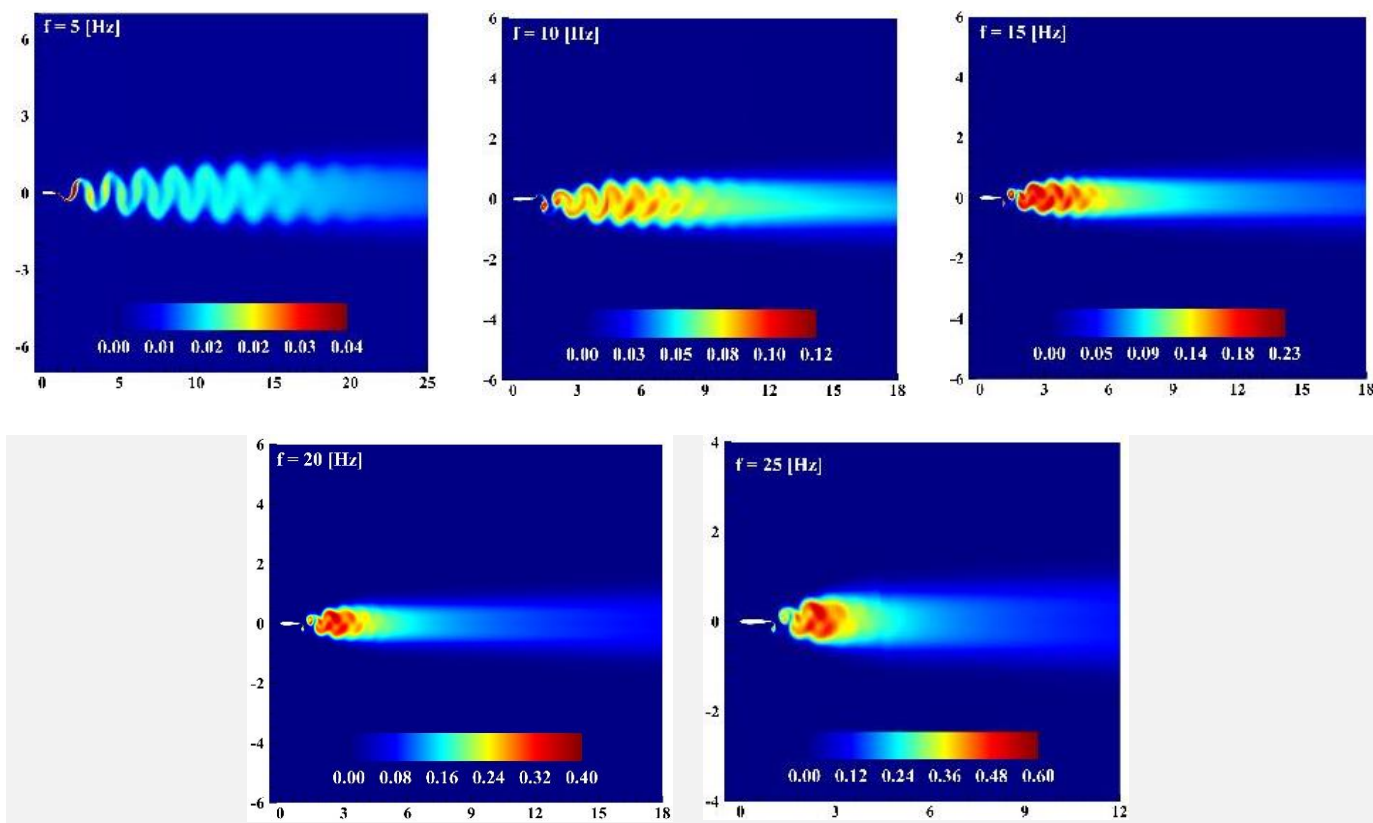
شکل ۷. خطوط هم‌مرز شدت آشفتگی جریان برای مدل پایه ایرفویل ناکا ۰۰۱۲ در فرکانس‌های چرخش به ترتیب از چپ به راست ۵، ۱۰، ۱۵، ۲۰ و ۲۵ هرتز.
