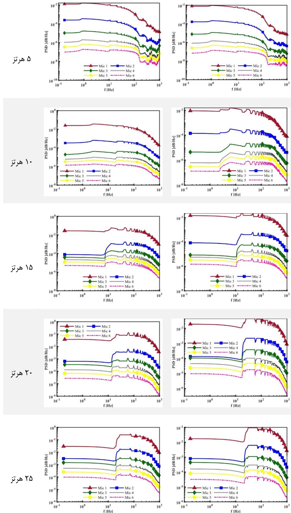
شکل ۱۲. مقایسه توزیع میانگین نمودارهای چگالی طیفی توان بر حسب فرکانس جریان در تمام فرکانس‌های نوسان ایرفویل ناکا ۰۰۱۲. سمت چپ) مدل پایه و سمت راست) مدل با دندان.
