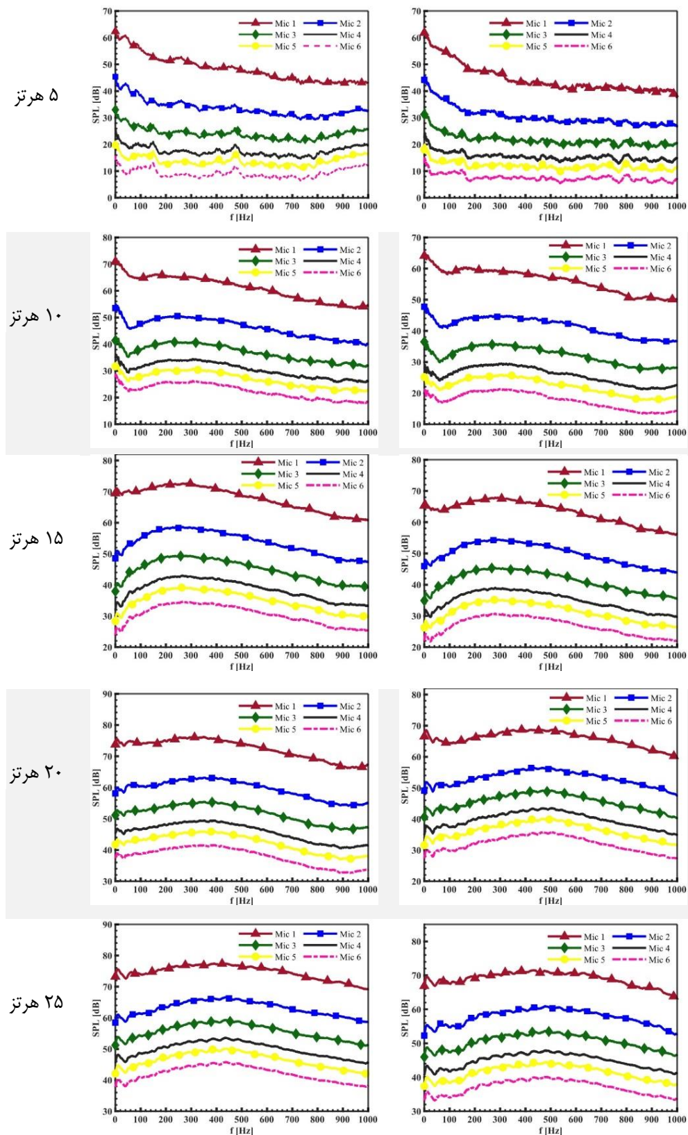
شکل ۱۳. مقایسه نمودارهای سطح فشار صوت بر حسب فرکانس جریان در تمام فرکانس‌های چرخش ایرفویل ناکا ۰۰۱۲. سمت چپ) مدل پایه و سمت راست) مدل با دندانه .
