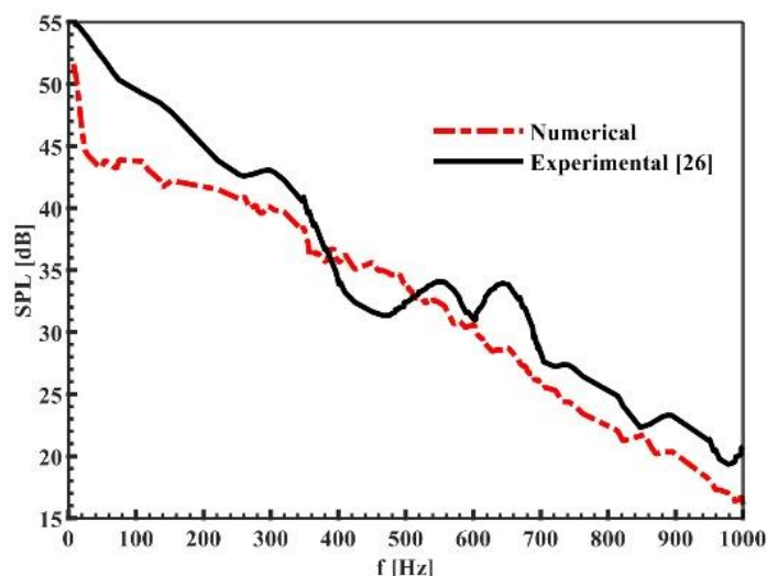
شکل ۶. ارزیابی نتایج اعتبارسنجی شبیه‌سازی پژوهش حاضر با نتایج تجربی مرجع [۲۶] برای سطح فشار صوت.
