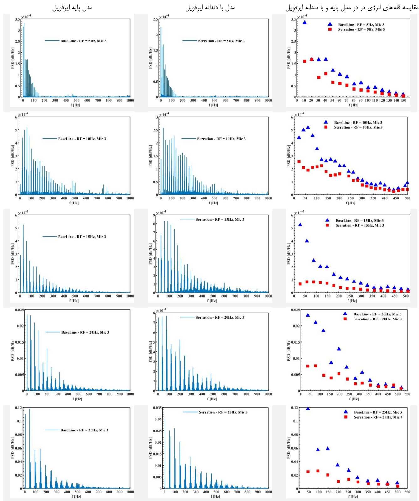
شکل ۱۱. نمودارهای چگالی طیف توان صوتی بر حسب فرکانس جریان همراه با مقادیر بیشینه در هارمونیک‌های فرکانس چرخش مرجع، برای دو مدل پایه و با دندانه ایرفویل ناکا ۰۰۱۲ در تمام فرکانس‌های چرخش ایرفویل و در فاصله ۱۰C.
