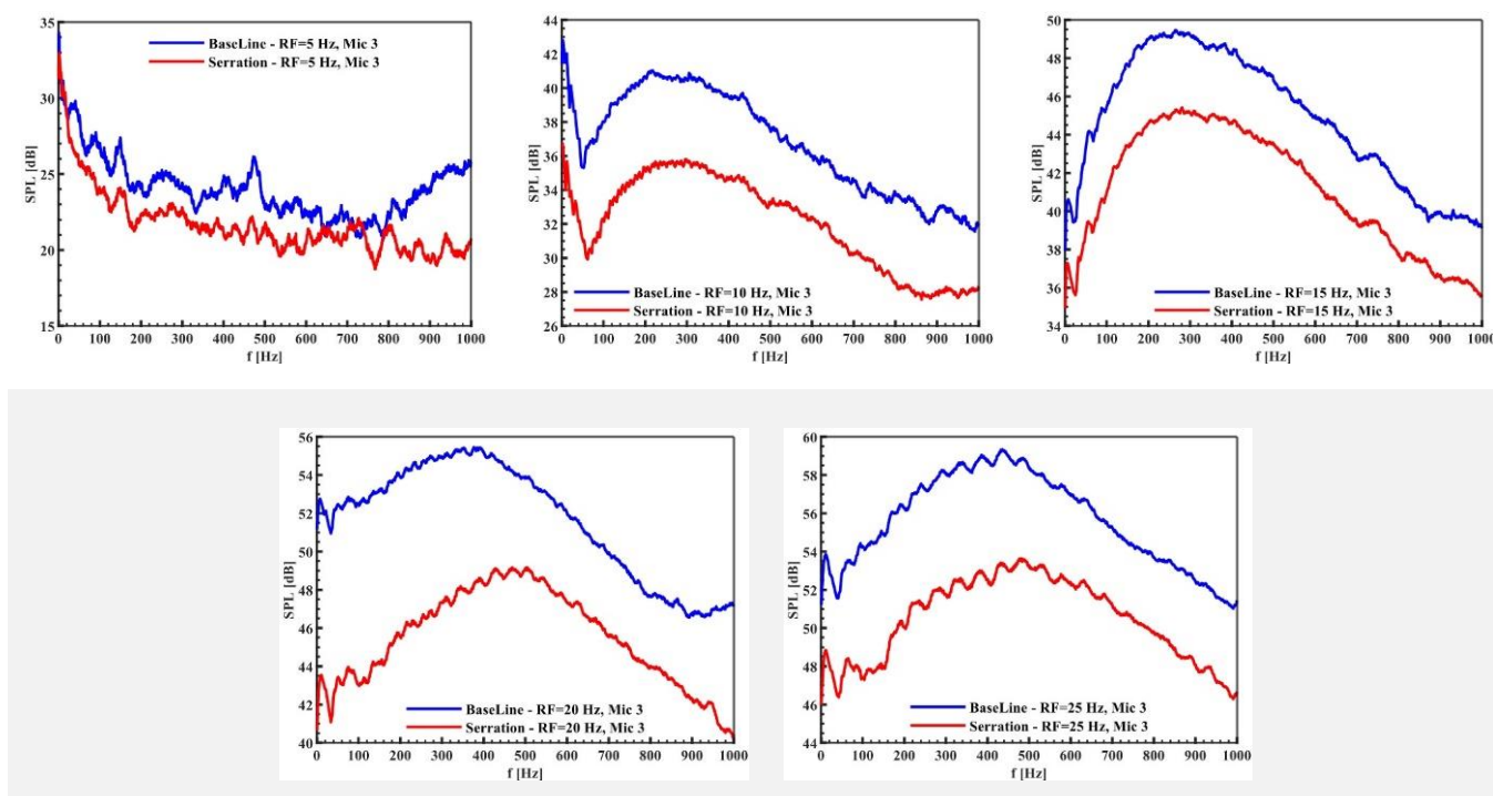
شکل ۱۵. مقایسه نمودارهای سطح فشار صوت بر حسب فرکانس جریان برای دو مدل پایه و با دندان ایرفویل ناکا ۰۰۱۲ در تمام فرکانس‌ها و فاصله 10C .
