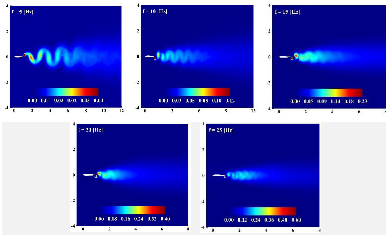
شکل ۸. خطوط هم‌مرز شدت آشفتگی جریان برای مدل با دندانه ایرفویل ناکا ۰۰۱۲ در فرکانس‌های چرخش به ترتیب از چپ به راست ۵، ۱۰، ۱۵، ۲۰ و ۲۵ هرتز.
