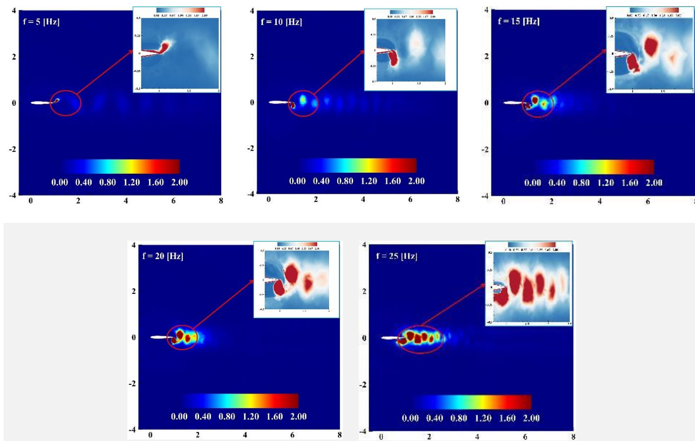
شکل ۱۰. خطوط هم‌مرز چرخش بی‌بعد برای مدل با دندان ایرفویل ناکا ۰۰۱۲ در فرکانس‌های چرخش به ترتیب از چپ به راست ۵، ۱۰، ۱۵، ۲۰ و ۲۵ هرتز.
