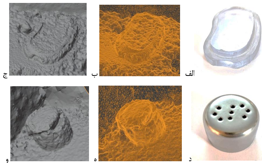
شکل ۱۱. فوتوگرامتری از قطعه‌ی شفاف و استیل، الف) قطعه شفاف، ب) مدل مش بندی قطعه شفاف، ج) مدل سه بعدی قطعه شفاف، الف) قطعه استیل، ب) مدل مش بندی قطعه استیل، ج) مدل سه بعدی قطعه استیل.
