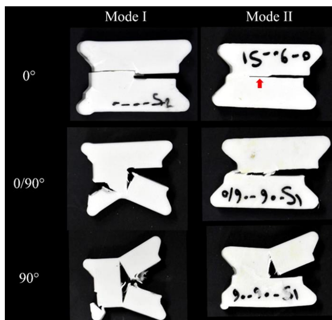
شکل ۱۱. تصاویر پس از شکست نمونه‌های چاپ‌شده در زوایای ۰°، ۹۰°/۰° و ۹۰° تحت مودهای شکست یک (کششی) و دو (برشی).
