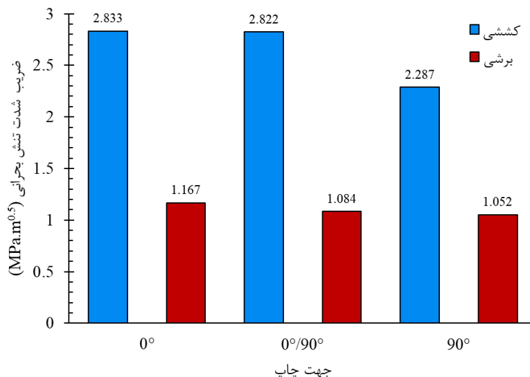
شکل ۹. مقادیر ضرایب شدت تنش بحرانی نمونه‌های ساخته شده به روش فیلامنت ذوب‌شده تحت نیروهای کششی و برشی با راستاهای ساخت ۰°، ۹۰° و ۰°/۹۰°.
