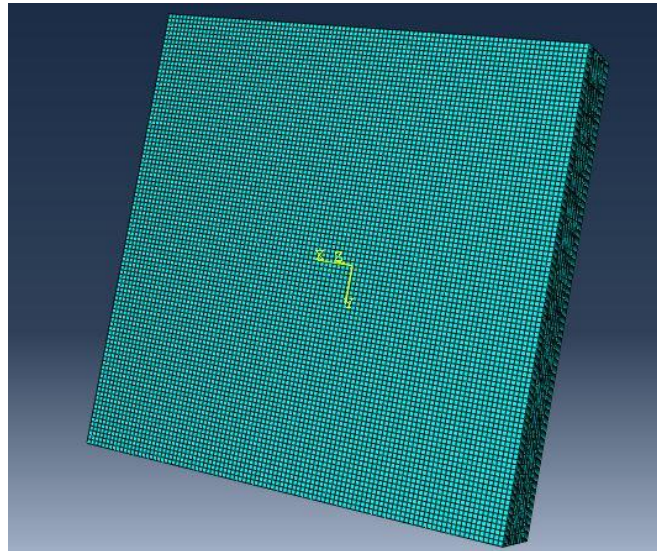
شکل ۲. تصویر شبکه‌بندی شده المان محدود ساندویچ پانل و عیوب صفحه‌ای
