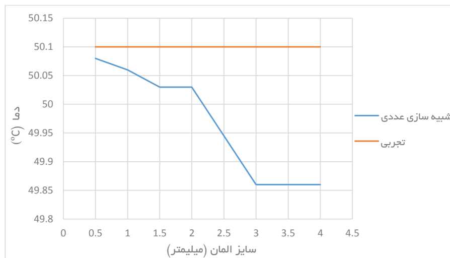
شکل ۳. نتایج همگرایی تحلیل اجزای محدود
