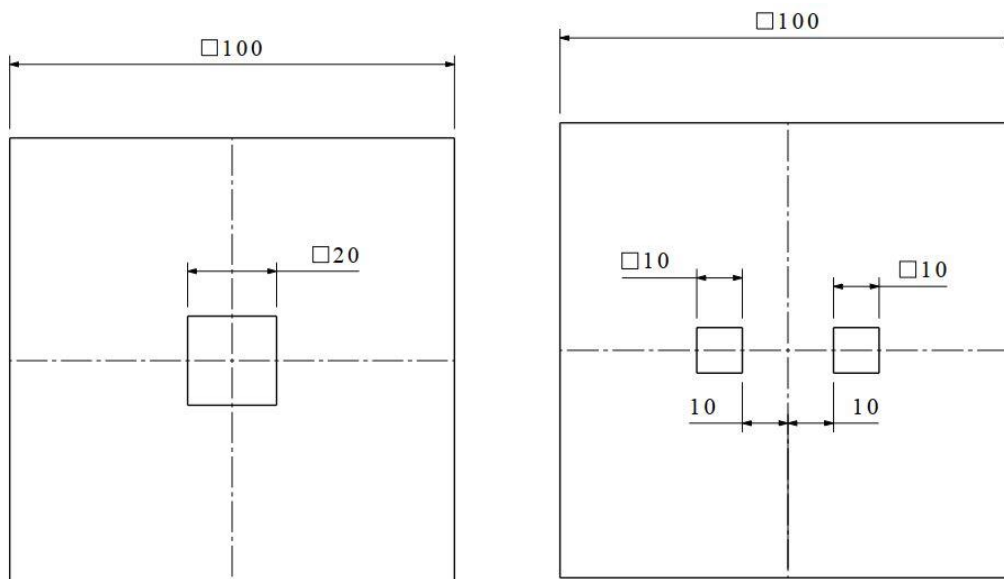
شکل ۱. تصویر شماتیک موقعیت قرارگیری عیوب
