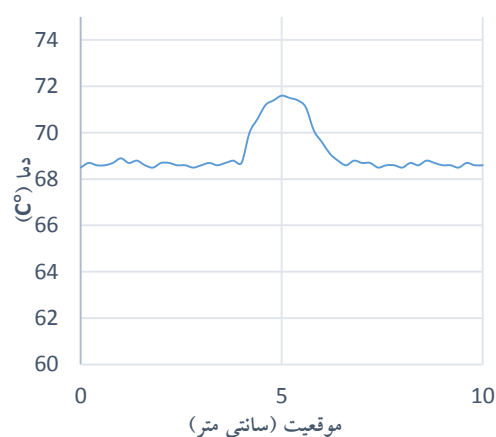
(ج) تغییرات دمایی سطح رویه نمونه 1D20
