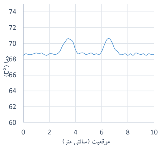
(د) تغییرات دمایی سطح رویه نمونه 2D10
