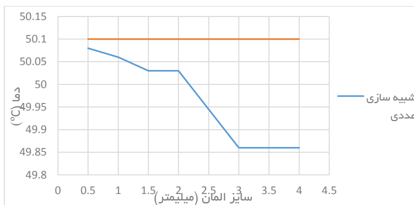
شکل ۳. نتایج همگرایی تحلیل اجزای محدود
