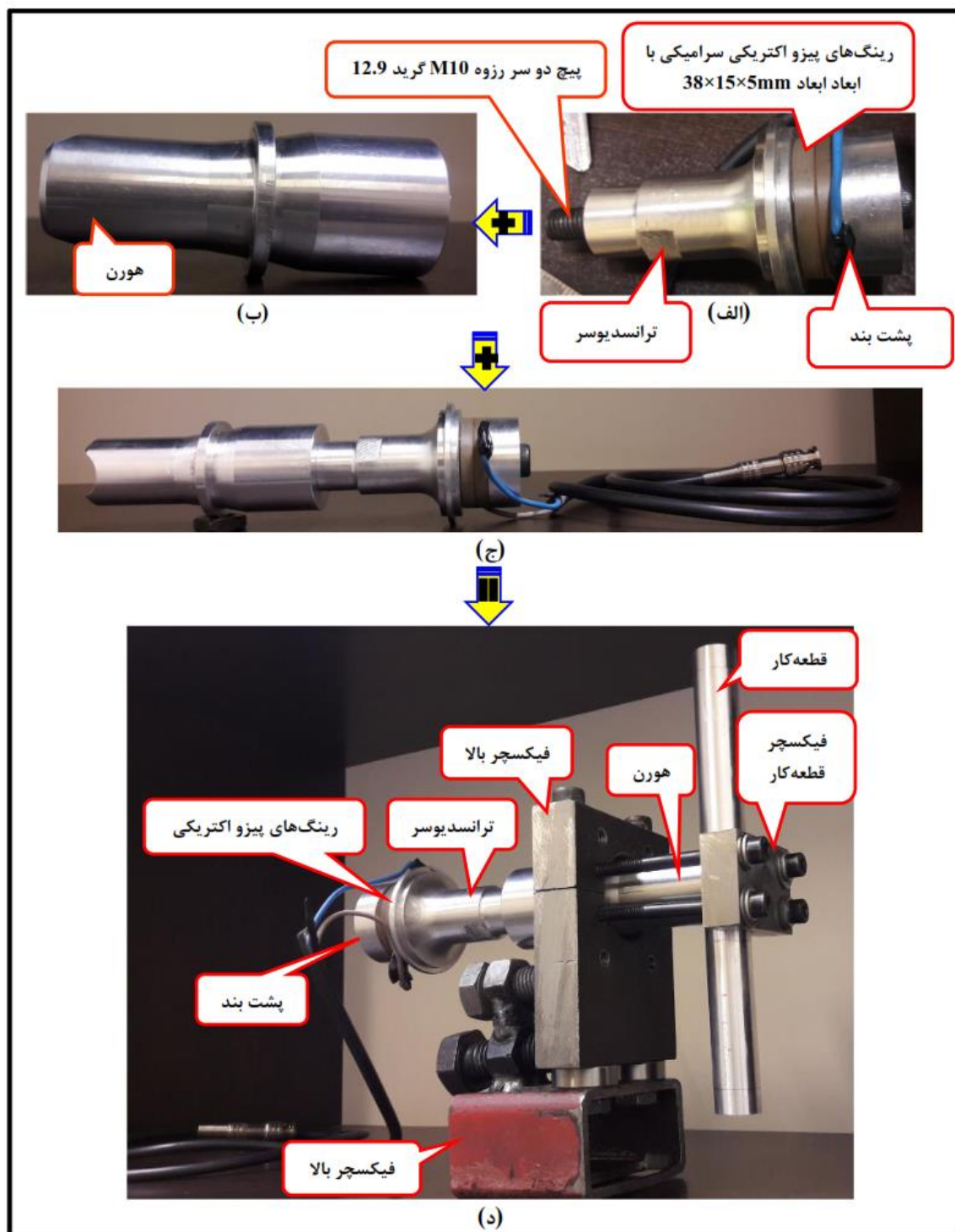
شکل ۲. چیدمان سیستم ارتعاشات فراصوت در فرآیند پرداخت کاری جریان ساینده مگنتورئولوژیکیال: الف) مونتاژ اجزای ترانسدیوسر شامل رینگ های پیزو الکتریک سرامیکی و پشت بند، ب) هورن فراصوت ساخته شده، ج) مونتاژ هورن فراصوت و ترانسدیوسر و د) مونتاژ سیستم فراصوت برای اعمال ارتعاشات به قطعه کار.
