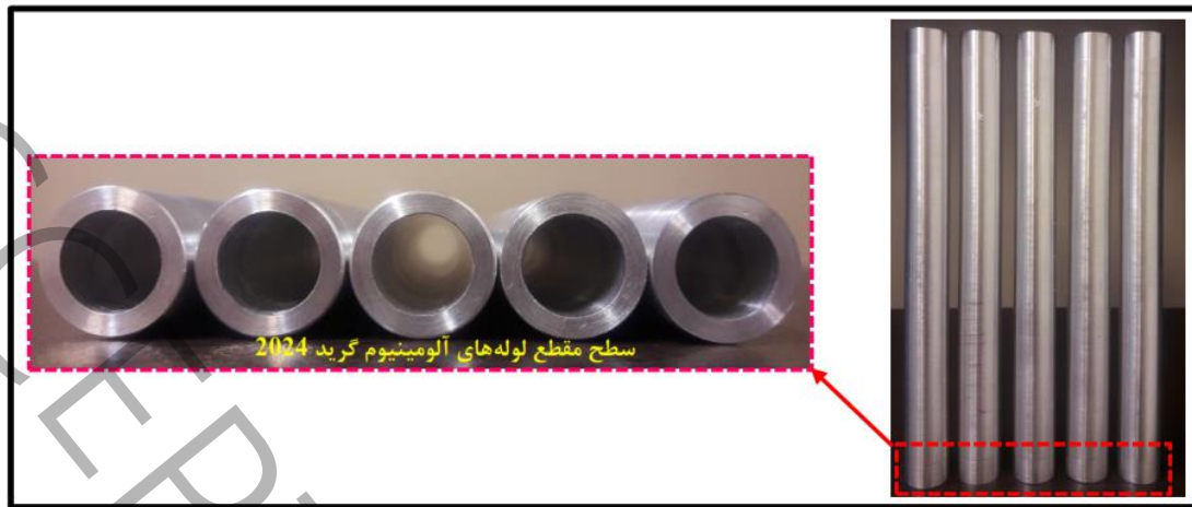
شکل ۶. تصاویر واقعی تعدادی از نمونه های لوله های آلایژ آلومینیوم ۲۰۲۴. Fig. 6. Actual images of a number of 2024 aluminum alloy tubes samples.
