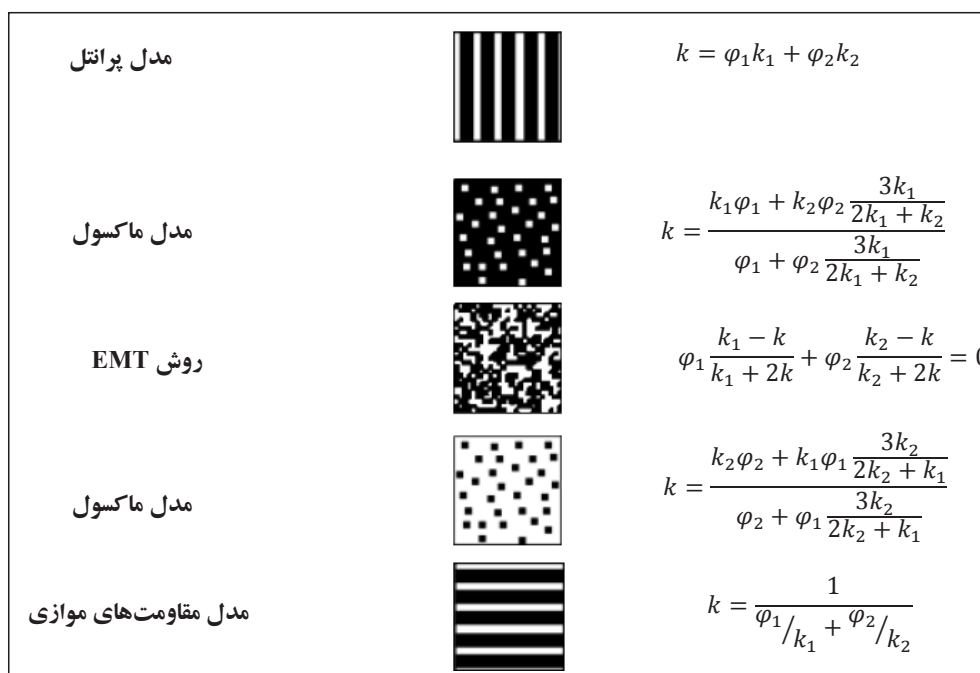
شکل ۶. پنج مدل مشهور برای تقریب ضریب انتقال حرارت مؤثر ترکیبات دوفازی [۳۱].
