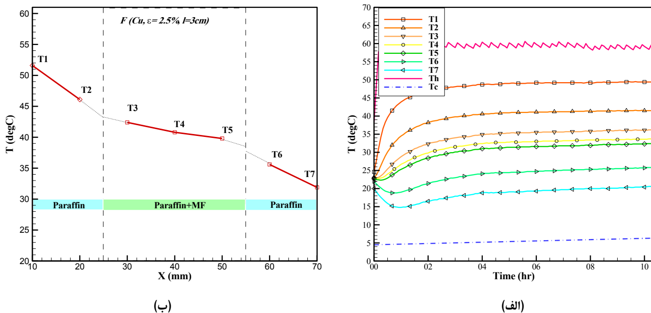
شکل ۸. (الف) تغییرات دمای وابسته به زمان (ب) توزیع دمای پایدار نمونه‌ی F.
