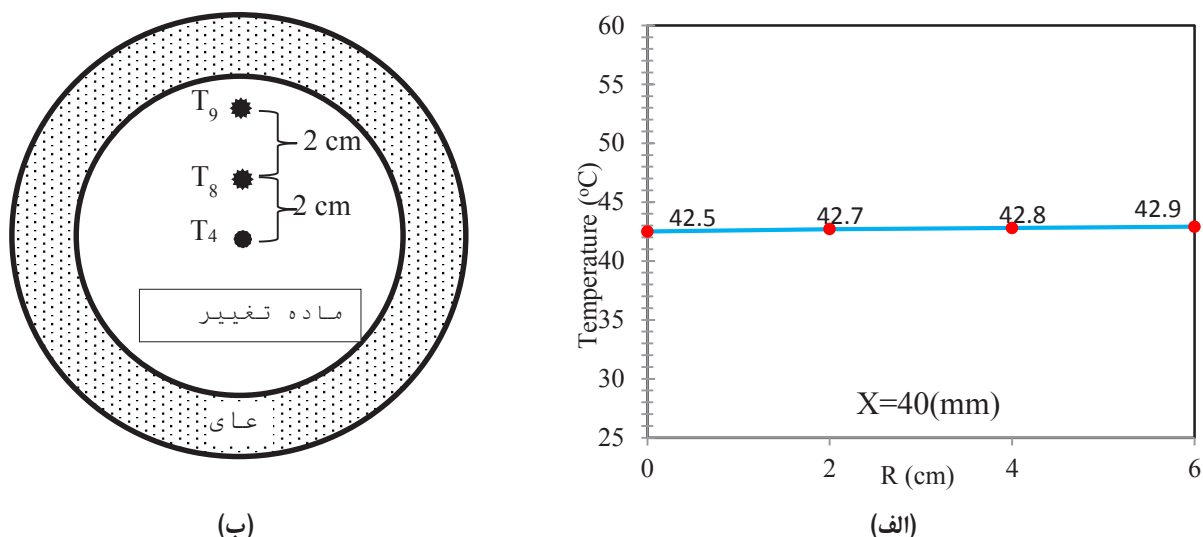
شکل ۳. (الف) توزیع دمای پایدار در راستای شعاعی استوانه (ب) طرح‌واره‌ای از چیدمان سنسورهای دما در راستای شعاعی
