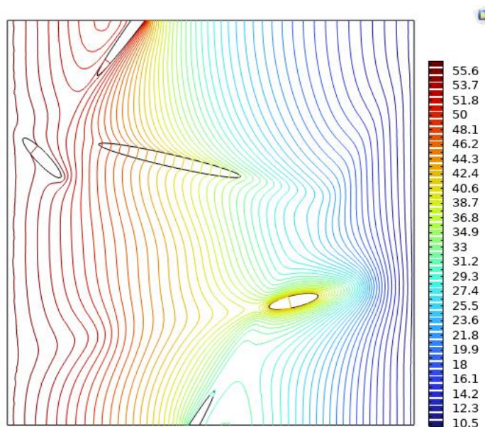
شکل ۱۱. توزیع دمای پایدار یک ترکیب دوفاز پارافین-الیاف فلزی در حالت جامد.
