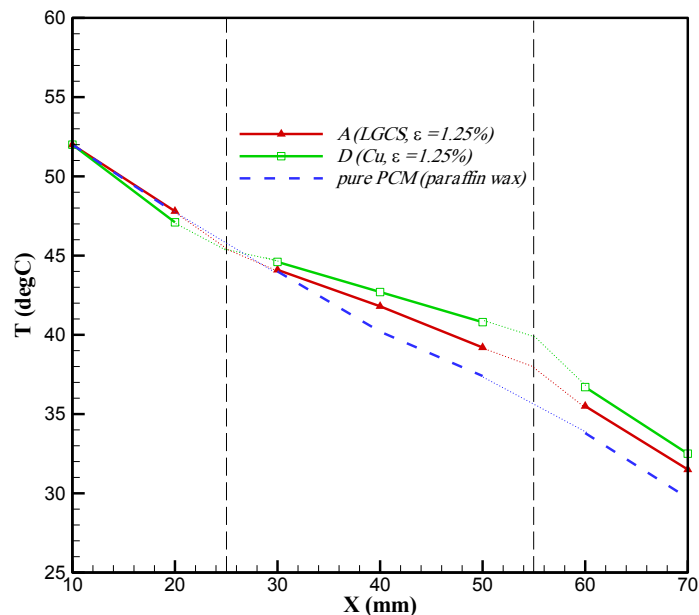
شکل ۹. مقایسه توزیع دمای پایدار در نمونه‌های A (الیاف استیل)، D (الیاف مسی) و پارافین خالص تحت شرایط یکسان.
