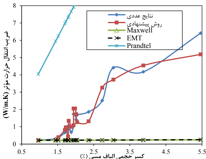
شکل ۱۴. مقایسه‌ی نتایج حل عددی با فرمول پیشنهادی و سایر مدل‌های تحلیلی برای محاسبه‌ی ضریب انتقال حرارت مؤثر ترکیب دوفازی.
