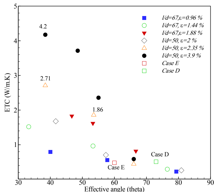
شکل ۱۳. بررسی عددی تغییر ضریب انتقال حرارت مؤثر ترکیب دو فاز یالیاف مسی-پارافین با تغییرات زاویه مؤثر و کسر حجمی یالیاف.
