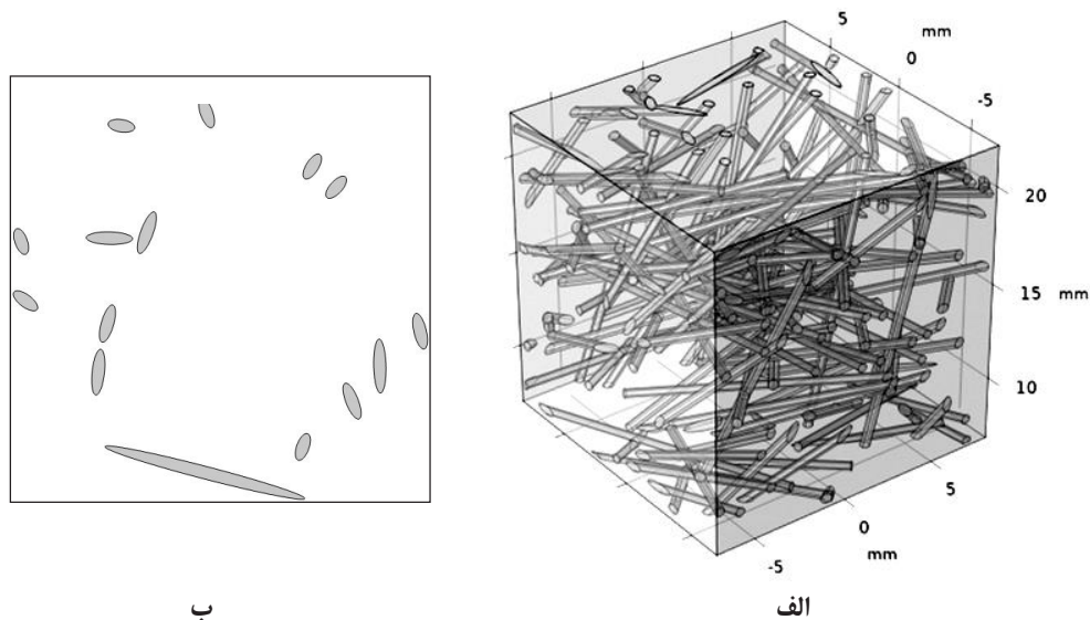
شکل ۵. (الف) برشی مکعبی از مدل عددی شامل الیاف فلزی و ماده تغییر فاز دهنده (ب) سطح مقطع الیاف در راستای عمود بر انتقال حرارت.
