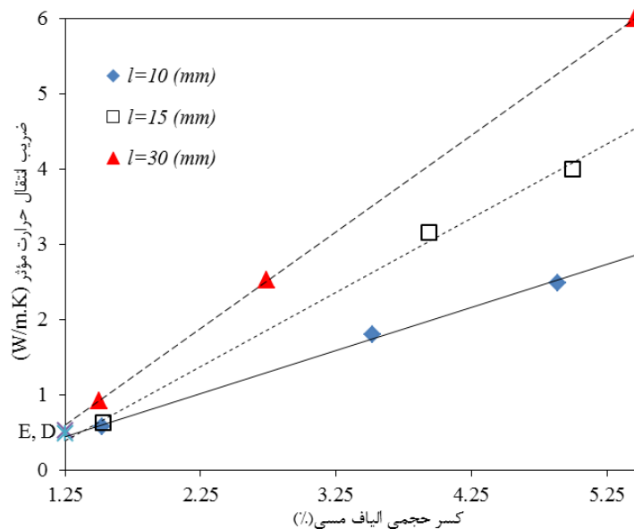
شکل ۱۰. تأثیر طول و کسر حجمی الیاف مسی بر ضریب انتقال حرارت مؤثر ترکیب دوفاز الیاف فلزی و پارافین ( d = 0.15 mm).
