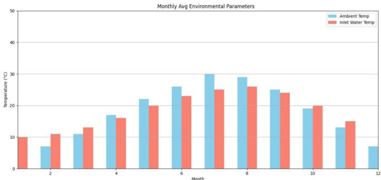
شکل ۹. عملکرد سالانه
