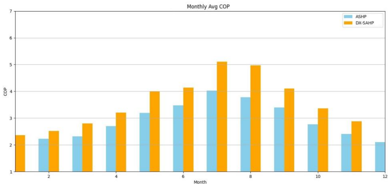
شکل ۱۰. عملکرد COP
