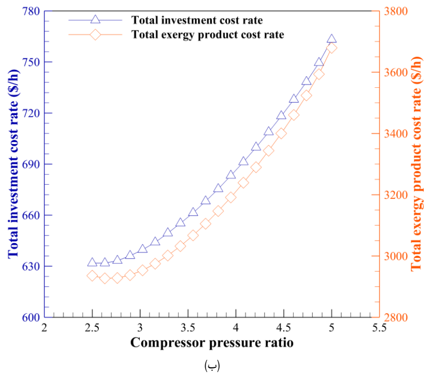
شکل ۵. نمودار تأثیر تغییرات نسبت فشار کمپرسورهای sCO_2 بر متغیرهای اصلی (الف) sCO_2 ، (ب) کل سامانه
