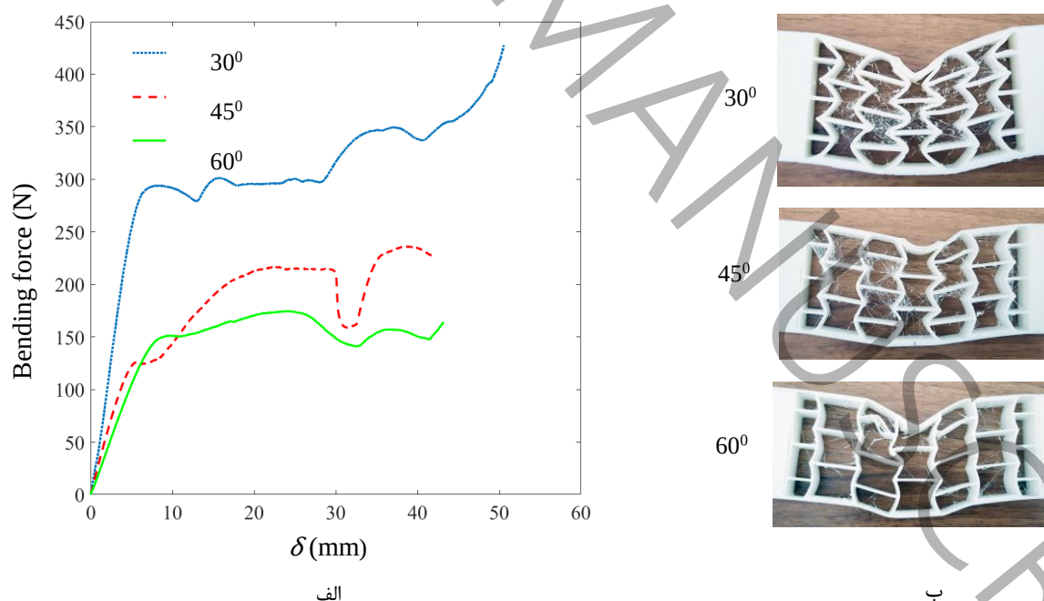
شکل ۷: الف) منحنی نیروی خمشی-جابجایی تیر و ب) نمونه‌های تیر ساندویچی با هسته آگزتیک دوبعدی خمیده ری-اینترنت شامل زوایای ۳۰، ۴۵ و ۶۰ درجه پس از آزمایش خمش سه نقطه.
