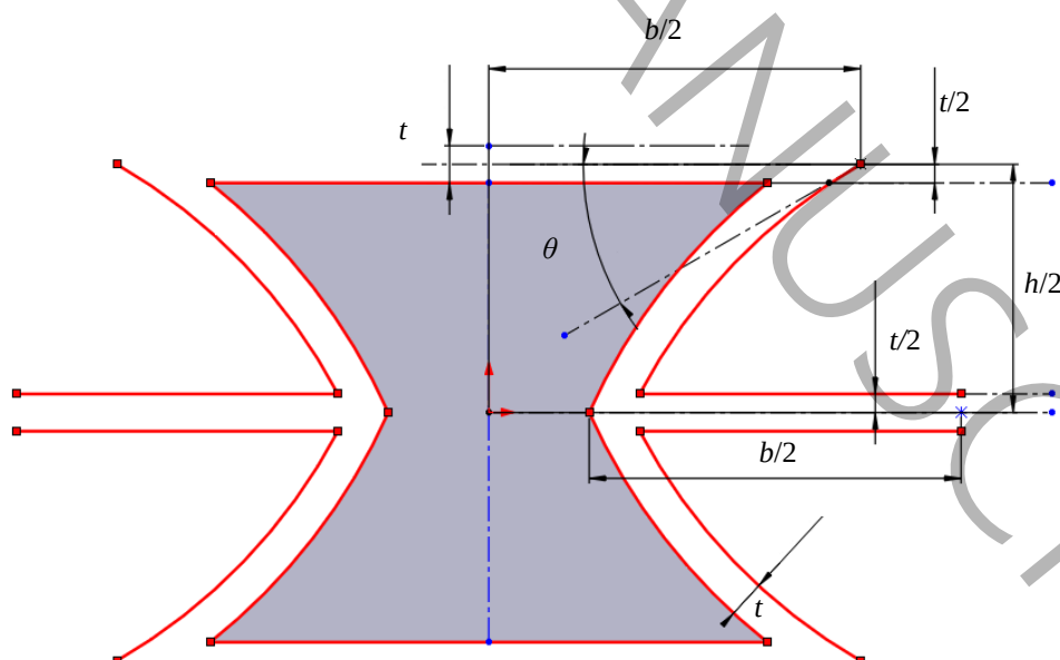
شکل ۲: شماتیک یک سلول واحد از هسته آگزتیک دوبعدی خمیده ری-اینترنت (با رنگ قرمز مشخص شده است).
