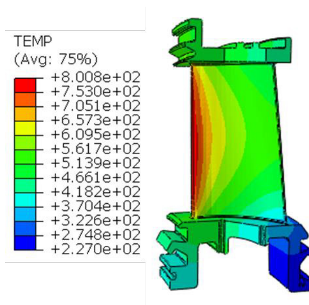
شکل ۴. توزیع دما در شرایط خستگی هم‌فاز و غیرهم‌فاز.
