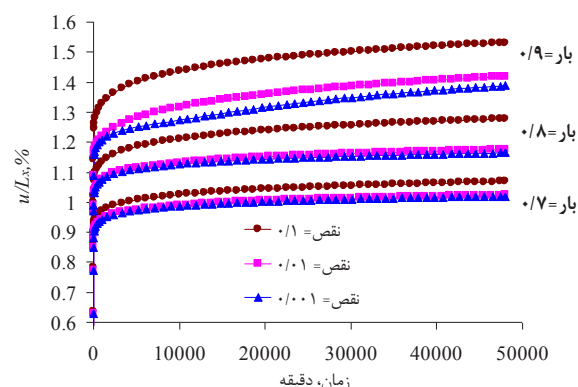
شکل ۱۲. منحنی کاهش طول ورق مستطیلی [۰/۹۰] ۲s با
