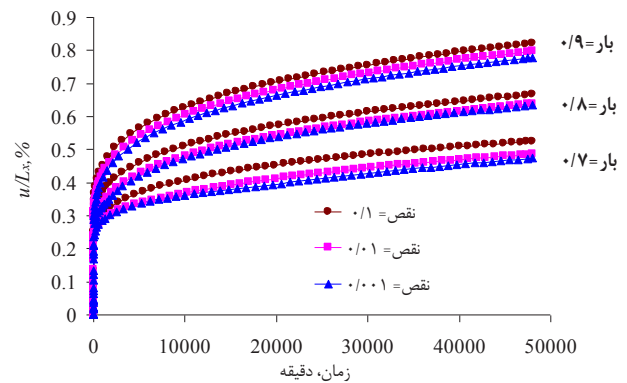
شکل ۸. منحنی کاهش طول ورق مستطیلی [45/-45]_4 با
