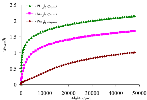
شکل ۱۰. منحنی خیز بی بعد ورق مستطیلی [۴۵ / -۴۵]۴ با نقص اولیه N_{0\epsilon} = ۷/۶۴۸ و ۰/۰۱
