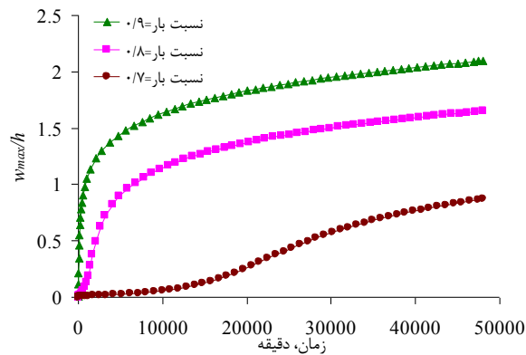
شکل ۹. منحنی خیز بی بعد ورق مستطیلی [۴۵ / -۴۵]۴ با نقص اولیه N_{0\epsilon} = ۷/۶۴۸ و ۰/۰۰۱
