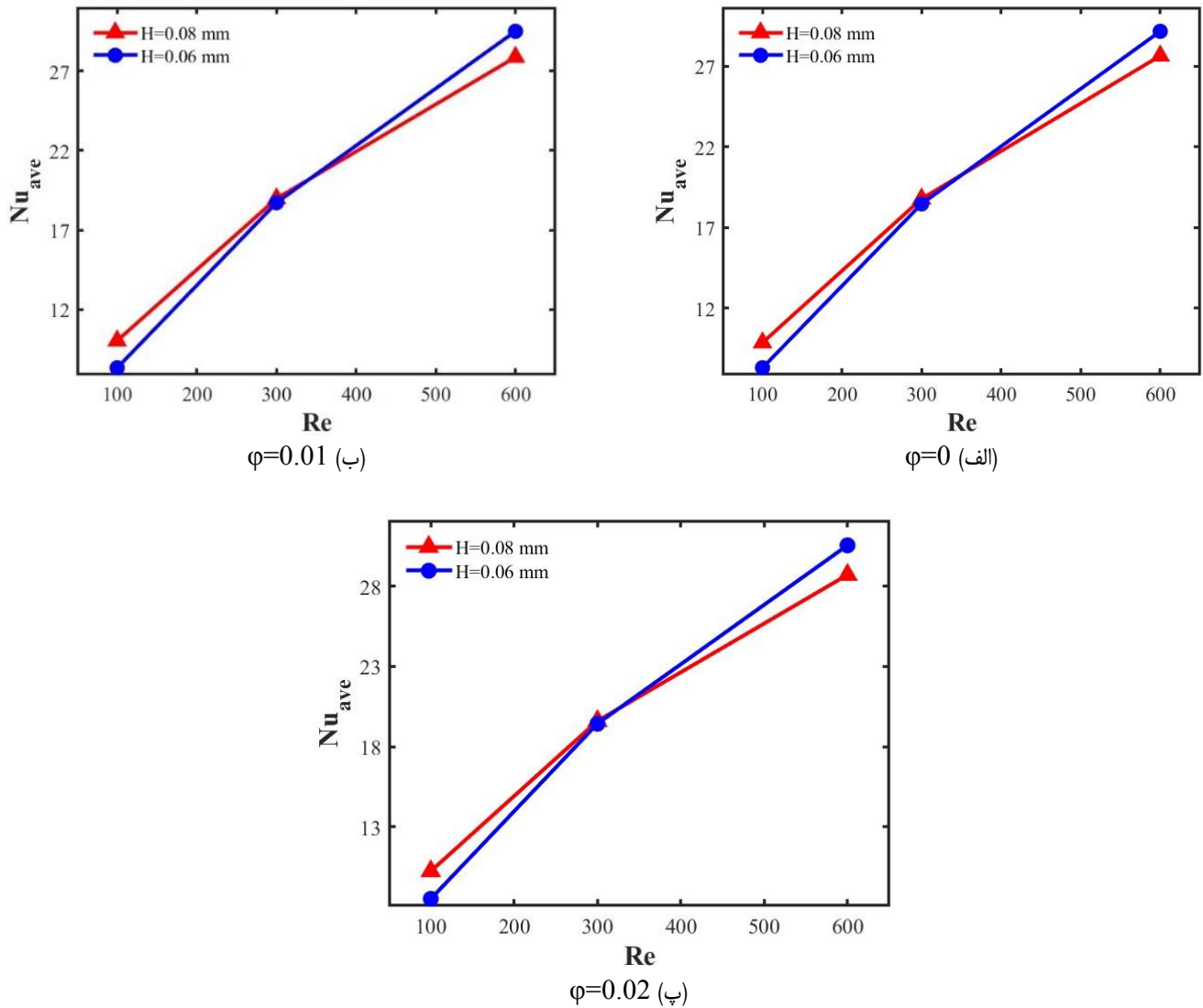
شکل ۱۷. تاثیر ارتفاع پره‌های منقطع مثلثی بر عدد ناسلت در میکروکانال در سه کسر حجمی مختلف.
