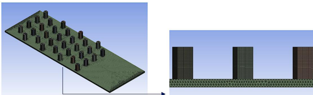
شکل ۴. نمای شماتیک شبکه‌بندی پژوهش حاضر
