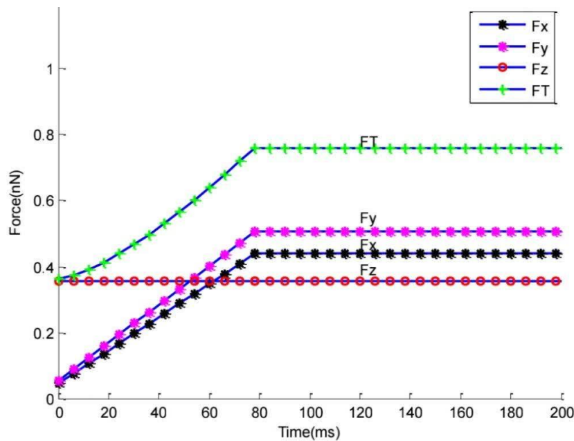
شکل ۳. نمودار نیروی منیپولیشن در راستاهای مختلف.
