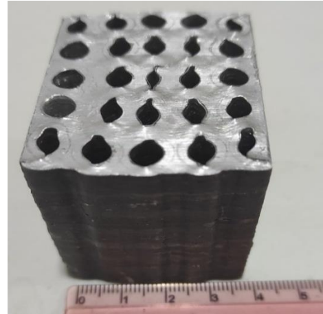
شکل ۳. شکل هندسی جاذب بعد از تغییر شکل و ایجاد تغییر شکل پلاستیک در آن.
