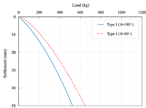
ب) تراکم نسبی ۵۵ درصد
