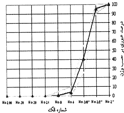
شکل (۲): منحنی دانه‌بندی درشت دانه
