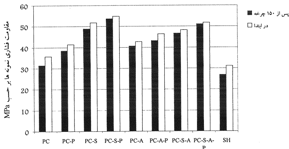
شکل (۴): مقایسه مقدار مقاومت فشاری نمونه‌ها در ابتدا و پس از ۱۵۰ چرخه یخبندان-نوب‌یخ.
