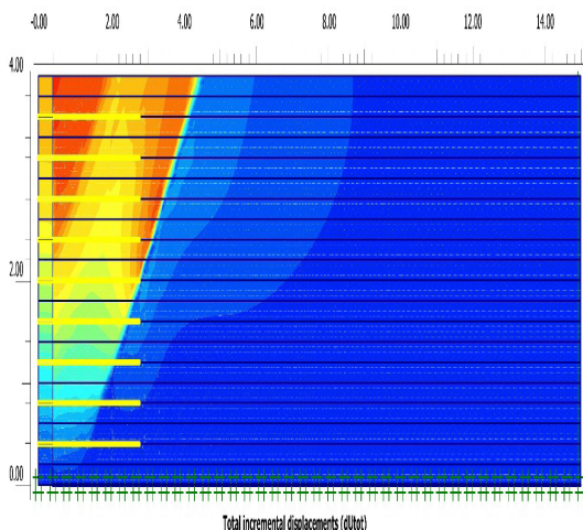
شکل ۶: گوهی گسیختگی الف) دیوار بر روی بستر صلب ب) دیوار بر روی بستر ضعیف Fig 6: Wedge failure. Right: Wall on rigid bed. Left: wall on poor floor
