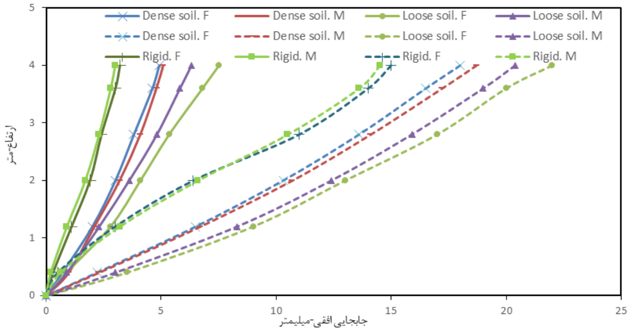
شکل ۱۳. جایجایی جانبی نمای دیوار در بررسی ترکیبی نوع اتصال ژئوگرید و شرایط بستر. خط ممتد: پایان ساخت. خط چین: سربار. Figure 14: Lateral displacement side view of the wall in the combined of the wall toe and bed conditions. Continuous line: rigid toe wall in finish condition. China Line: Free Tail.
