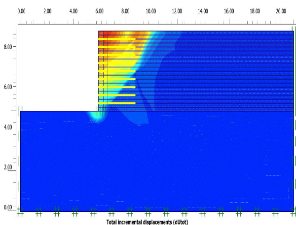
شکل ۶: گوهی گسیختگی الف) دیوار بر روی بستر صلب ب) دیوار بر روی بستر ضعیف Fig 6: Wedge failure. Right: Wall on rigid bed. Left: wall on poor floor
