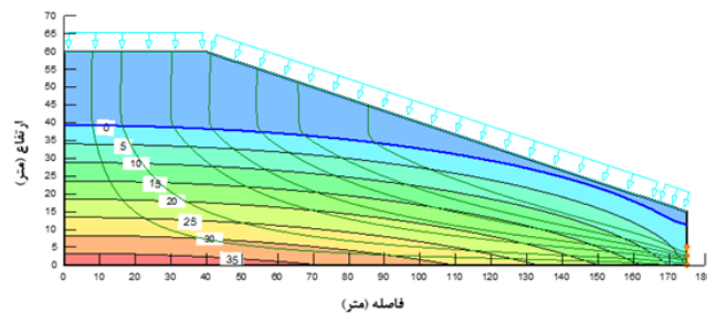
شکل ۹. منحنیهای هم‌فشار و خطوط جریان در خاک شیبدار بعد از ۴ روز بارندگی با شدت ۲/۸۸ میلی‌متر بر ساعت (سطح شیبدار بدون زهکش افقی است) Fig9. Pressure contours and flow lines in soil after 4 days of precipitation with intensity of 2.88mm/h (slope without any horizontal drainage)
