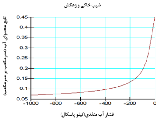
شکل ۷. تابع محتوای آب در مصالح شیب خاکی و زهکش افقی Fig7. Water content function in earthen slope and horizontal drainage materials
