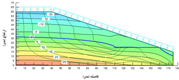
شکل ۱۰. منحنی‌های هم‌فشار و خطوط جریان در خاک شیبدار بعد از ۴ روز بارندگی با شدت ۲/۸۸ میلی‌متر بر ساعت (زهکش افقی در ارتفاع ۲۰ متری با طول ۵۰ متر و ضخامت ۱۰۰ میلی‌متر است) Fig10. Pressure contours and flow lines in soil after 4 days of precipitation with intensity of 2.88 mm/h (horizontal drainage with 20 m high, 50 m long and 100 mm thick)
