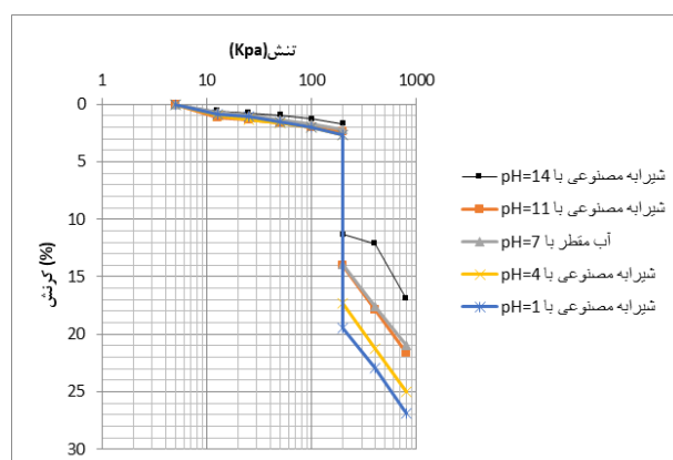
شکل ۴. نمودار مقایسه فروریزش خاک اشباع با شیرابه با pH های مختلف
