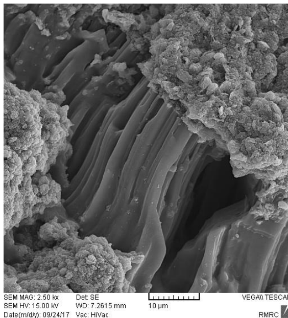
شکل ۲۶. تصویر میکروسکوپ الکترونی نمونه خاک حاوی شیرابه با بزرگنمایی ۲۵۰۰ برابر SEM image of a soil contaminated with lea-chate with a magnification of 2500 times
