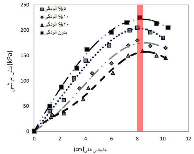
شکل ۲۲. منحنی برشی خاک CL (۹۶ ساعته) (۱۰۰ kPa) Shear curve of CL (96 hours) (100kPa)
