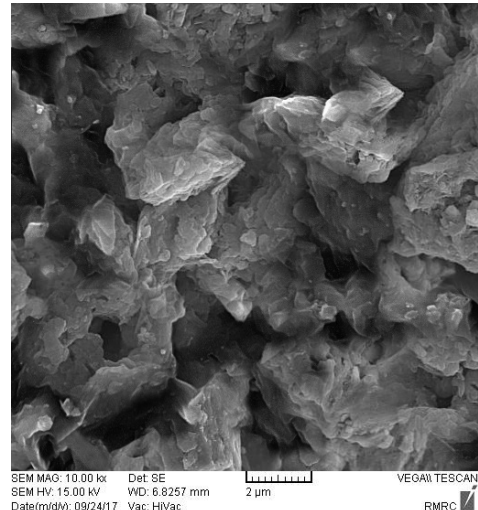
شکل ۹: تصویر میکروسکوپ الکترونی نمونه خاک حاوی شیرابه با بزرگنمایی ۱۰۰۰۰ برابر SEM image of a soil contaminated with lea-chate with a magnification of 10000 times
