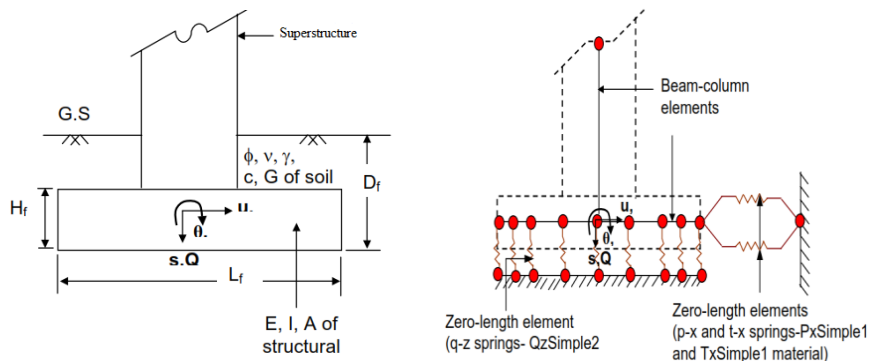
شکل ۵. مدل BNWF برای فونداسیون های سطحی [۲] Fig. 5. Schematic diagram of the proposed BNWF model for shallow foundations
