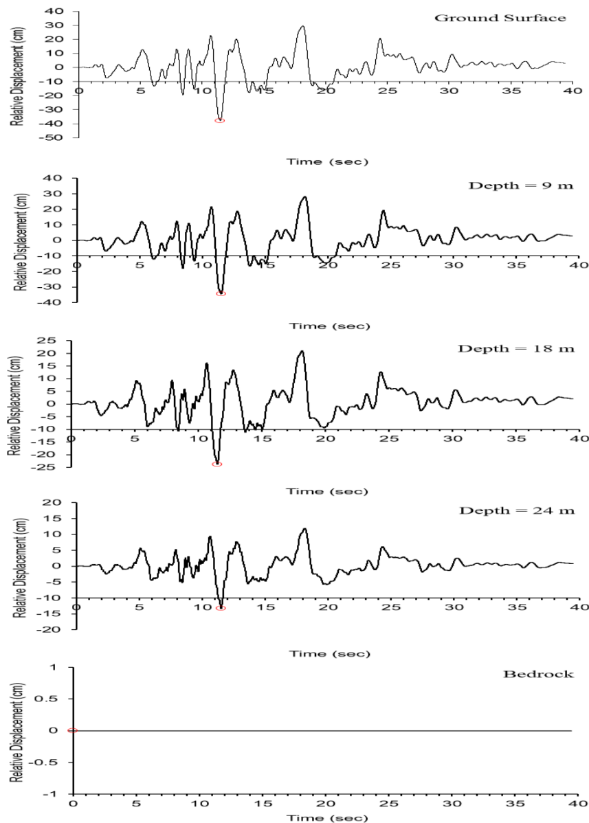
شکل ۷. پاسخ اثر ساختمان بر جابجایی زلزله ی Loma Prieta در مدل واقع بر خاک نوع IV
