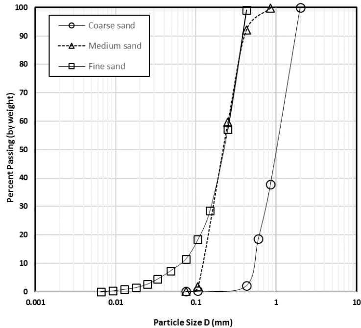
شکل ۴. منحنی دانه‌بندی خاک‌های مورد مطالعه Fig. 4. The grading curve of studied soils
