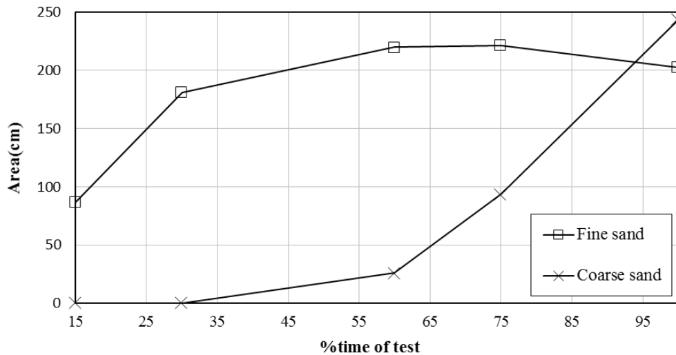
شکل ۱۲. مساحت توده آلودگی در بازه‌های زمانی مختلف در دو خاک در نمونه ریزدانه به درشت‌دانه
