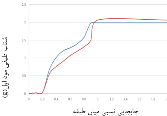
شکل ۱۷. مقایسه منحنی میانه IDA قاب ستون-پیوند و قاب خمشی تحت اثر توالی لرزه‌ای در سطح عملکرد LS Fig. 17. Median IDA curve considering MS-AS effect for Moment Frame and Linked-Column Frame in LS performance level
