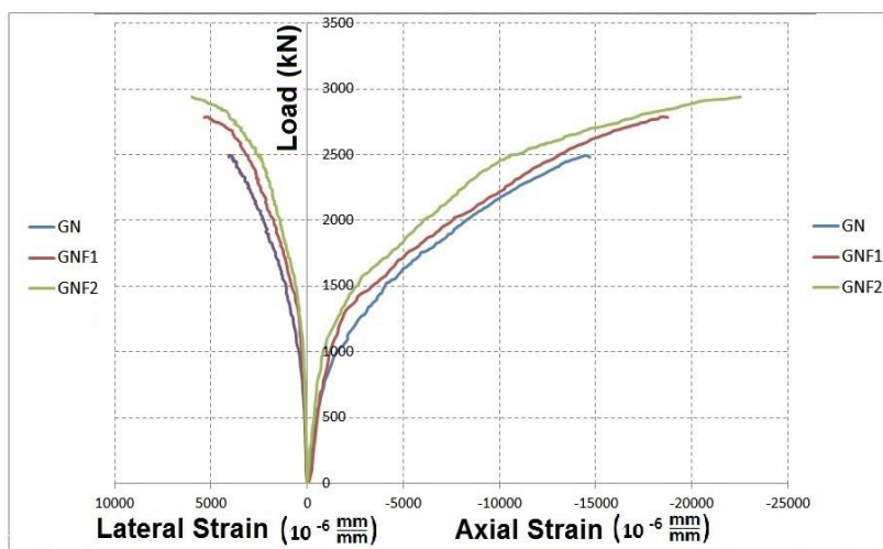
شکل ۱۱. منحنی بار-کرنش برای ستون های دارای غلاف GRP Fig. 11. Load-strain curve for columns with GRP casing
