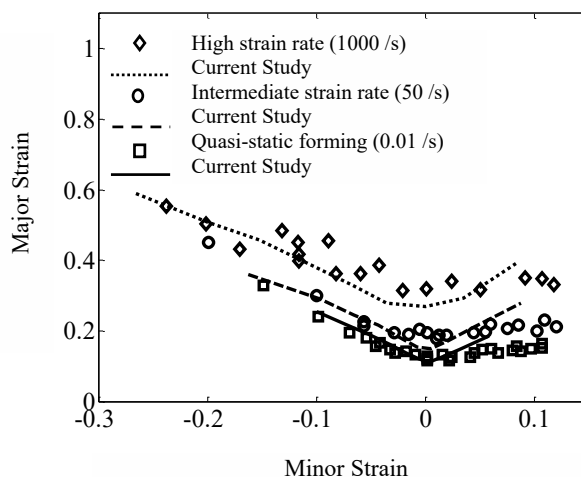
شکل ۳: مقایسه نتایج عددی پاسخ به نرخ کرنش برای آلیاژ ۶۰۶۱-T۶ با نتایج تجربی دریانی و همکاران [۸]
