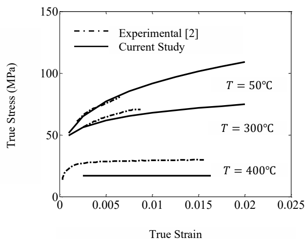
شکل ۲: مقایسه نتایج عددی پاسخ تنش-کرنش آلیاژ AA ۳۱۰۴ با نتایج تجربی ون هافتن و همکاران [۲]
