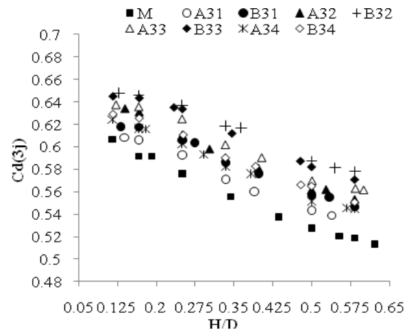
شکل ۹. تغییرات ضریب دبی نسبت به عمق استغراق با ۳ گردابشکن هرمی
