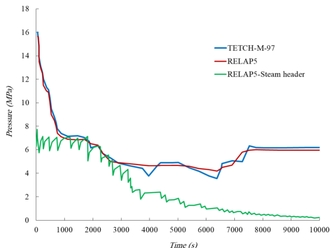
شکل ۸: تغییرات فشار خروجی راکتور و خط بخار در طی شکست ۲۵ میلی متر
