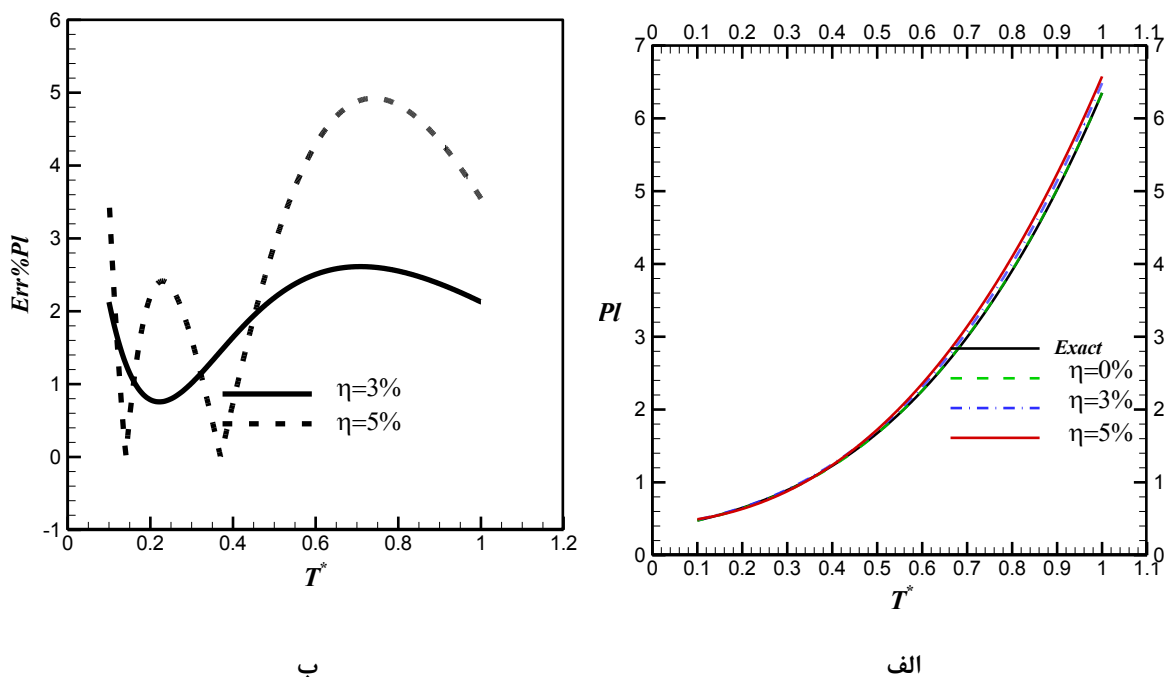
شکل ۶: نتایج بازسازی هدایت پذیری مورد شماره دو الف) نمودار توزیع پلانک برای ۳ حالات دقیق و بازسازی شده با سه خطای ۰، ۳ و ۵ درصد ب) نمودار توزیع خطای نسبی عدد پلانک پس از بازسازی برای خطای اعمالی ۳ و ۵ درصد
