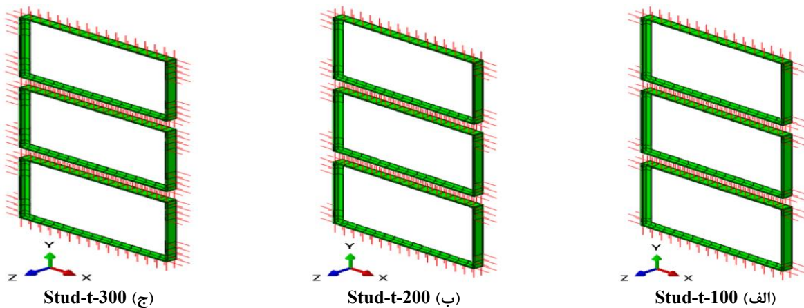
شکل ۸. نمای سه بعدی اتصال گل میخ (Stud) با قرار گیری گل میخ در طول (الف) ۱۰۰ (ب) ۲۰۰ (ج) ۳۰۰ میلی متر از دو انتهای ستون Fig. 8. 3D view of Stud connection with placing of studs at length of (a) 100, (b) 200, (c) 300 mm from ends of column
