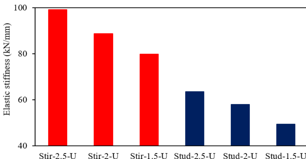
شکل ۲۳. مقایسه سختی الاستیک نمونه‌ها
