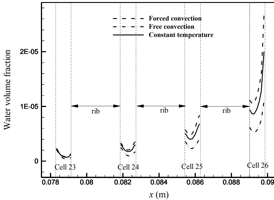
شکل ۹: کسر حجمی آب ورودی چهار سلول انتهایی
