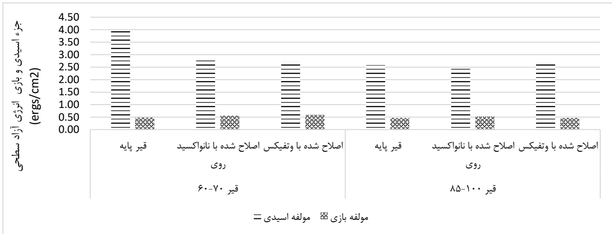
شکل ۸. مؤلفه های اسیدی و بازی انرژی آزاد سطحی (ergs/cm 2 ) Fig. 8. Acidic and basic component of surface free energy of asphalt binder (ergs/cm 2 )
