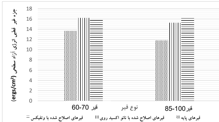
شکل ۹. جزء غیر قطبی انرژی آزاد سطحی قیرها ( \text{ergs}/\text{cm}^2 )
