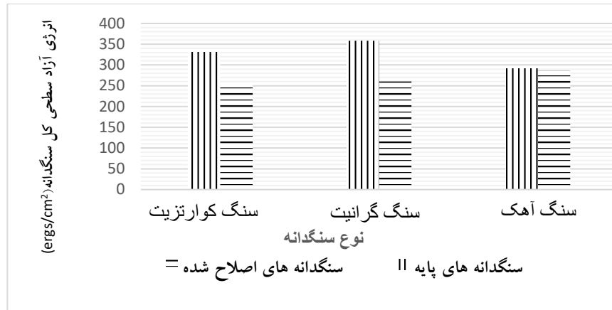
شکل ۱۰. انرژی آزاد سطحی کل سنگدانه ها ( \text{ergs}/\text{cm}^2 )
