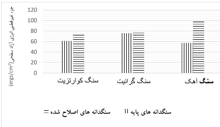
شکل ۱۳. جزء غیر قطبی انرژی آزاد سطحی سنگدانه ها ( \text{ergs/cm}^2 )
