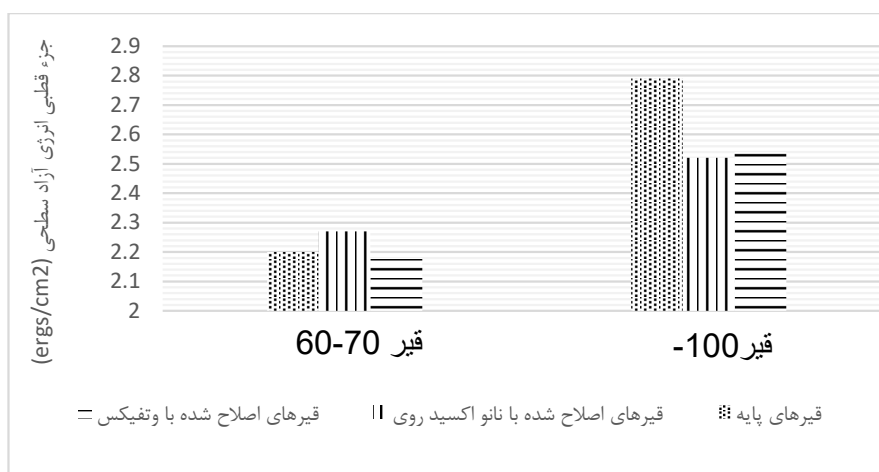
شکل ۷. جزء قطبی انرژی آزاد سطحی قیرها (ergs/cm²)
