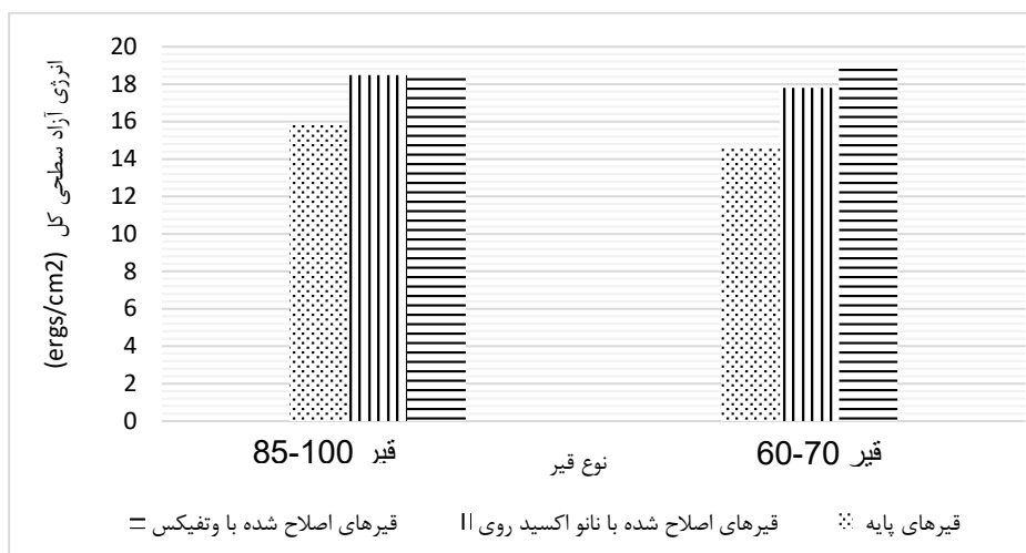
شکل ۶. انرژی آزاد سطحی کل قیرها (ergs/cm²)
