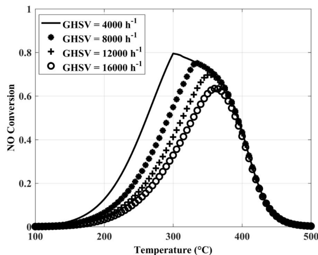
شکل ۲. تغییرات میزان تبدیل اکسید نیتروژن در دما و سرعت‌های حجمی متفاوت،
