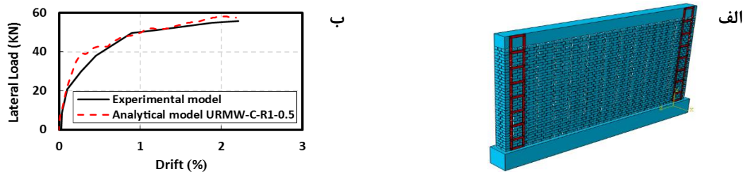
شکل ۱۳. الف) مدل سازی اجزا محدودی نمونه شاهد URMW-C-R1-0.5 ب) نمودار نیرو-جابجایی نمونه تحلیلی با نمونه شاهد آزمایشگاهی Fig. 13. a) Finite element model of reference specimen URMW-C-R1-0.5 b) Force-displacement curve of analytical specimen and experimental reference specimen.
