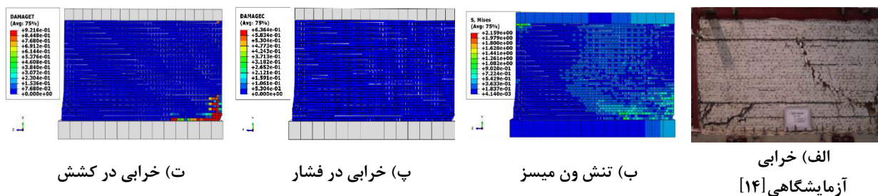
شکل ۱۰. خرابی نمونه شاهد آزمایشگاهی و نمونه تحلیلی URMW-C-0.5
