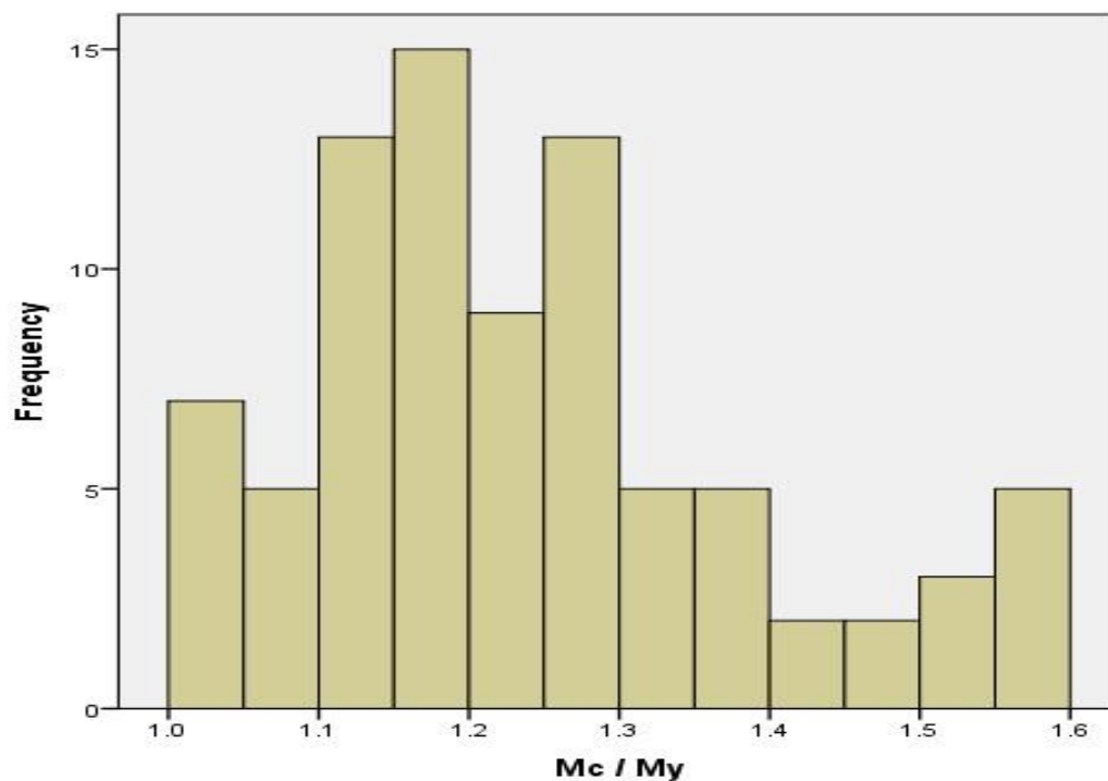
شکل ۱۹. هیستوگرام فراوانی پارامتر نسبت سختی بعد از نقطه‌ی تسلیم ( M_c / M_y ) برای دیوار برشی کوتاه
