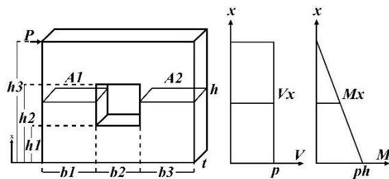
شکل ۱۰. شماتیک کلی از یک دیوار بنایی دارای بازشو و تلاش های ایجاد شده در ارتفاع دیوار
