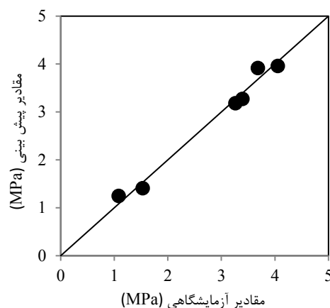
شکل ۷: مقایسه نتایج آزمایشگاهی و نتایج پیش بینی حاصل از رابطه پیشنهادی (۱)
