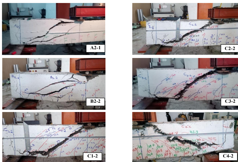
شکل ۵. مود خرابی در نمونه‌های تیر Fig. 5. Failure mode of beam specimens
