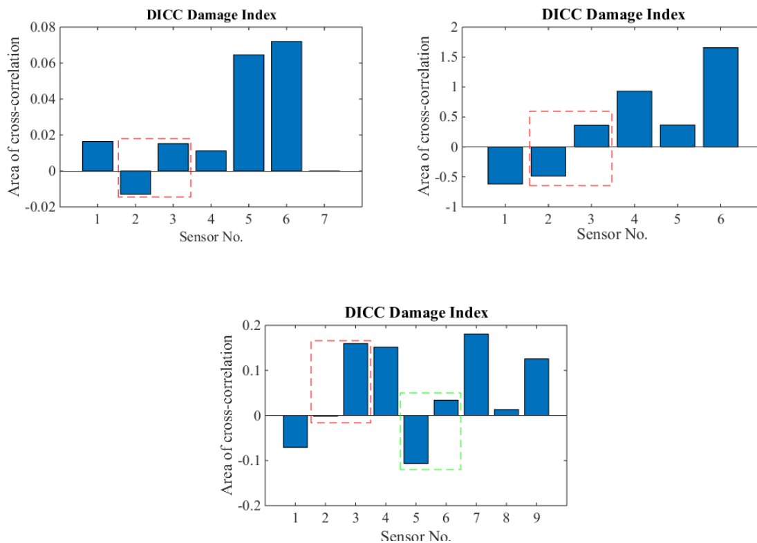
شکل ۶. شاخص آسیب DICC برای A) سناریوی آسیب یک، B) سناریوی آسیب دو و C) سناریوی آسیب چهار برای مقدار آسیب ۱۰٪/۱۰٪ Fig. 6. DICC Damage Index for A) Damage Scenario 1, B) Damage Scenario 2, C) Damage Scenario 4 for %10 damage value.
