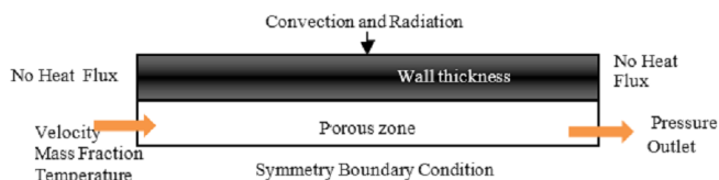
شکل ۱. هندسه مسئله به همراه شرایط مرزی
