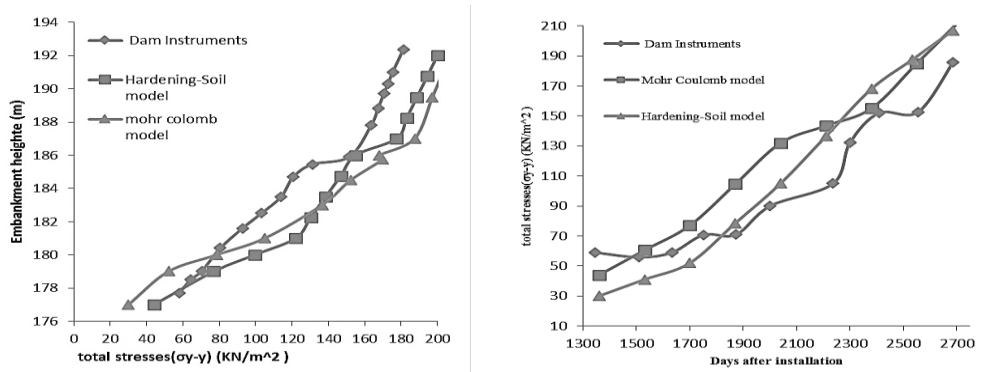
شکل ۸. وضعیت تغییرات تنش کل با زمان ساخت و ارتفاع خاکریزی مقطع ۱۹، ابزار دقیق و آنالیز برگشتی مدل HS
